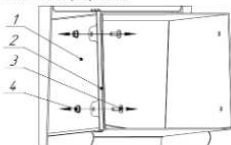
Рисунок 7 — Снятие кронштейна дверки (базовое расположение)
