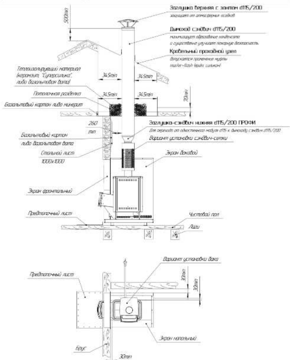
Рисунок 6 - Схема установки печи с защитными экранами
