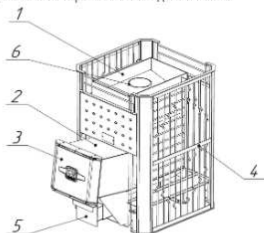
Рисунок 1б - Конструкция печи «ТАМАНЬ-СЕТКА (1.1)»
