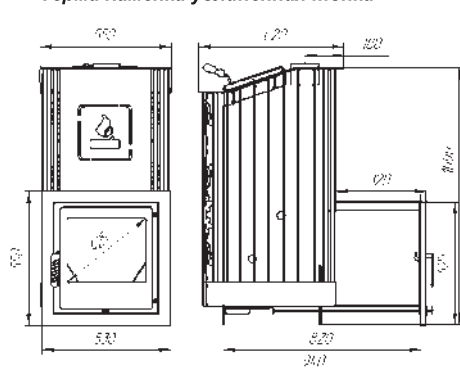
Терма Каменка удлиненная топка
