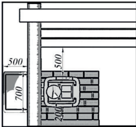
Безопасные расстояния вид сверху (рис.2)
