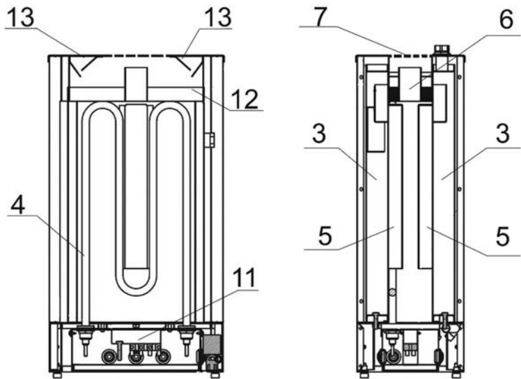
Рис.2 Устройство АЭПП
