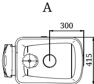
Рисунок 3. Габаритные размеры печи «Ангара 2012» с коротким топливным каналом
