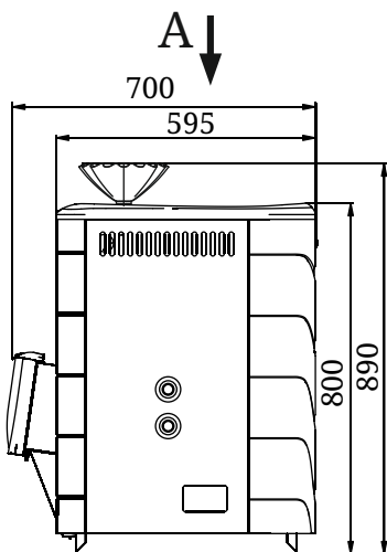
Рисунок 3. Габаритные размеры печи «Ангара 2012» с коротким топливным каналом
