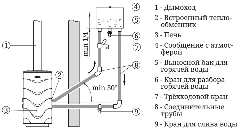
Рисунок 10. Схема монтажа системы водонагрева с использованием встроенного теплообменника
