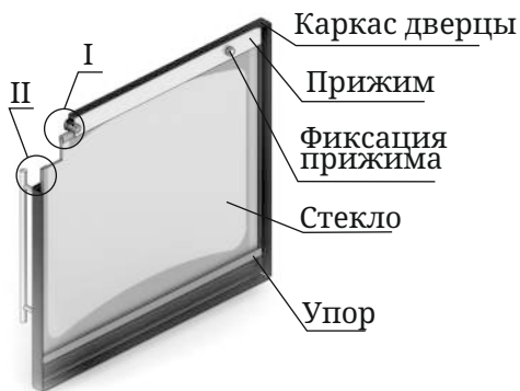
Рисунок 14. Ремонт светопрозрачного экрана дверцы модели «Витра»
