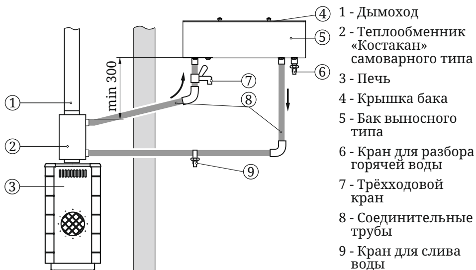
Рисунок 9. Схема монтажа системы водонагрева с использованием теплообменника «самоварного» типа
