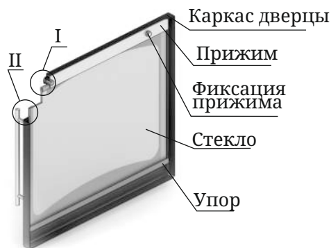
Рисунок 10. Ремонт светопрозрачного экрана дверцы модели «Витра»
