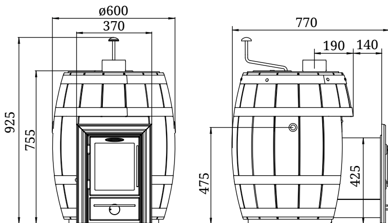
Рисунок 3. Габаритно-монтажные размеры печи-кондиционера модификация «Скоропарка 2012 Баррель»
