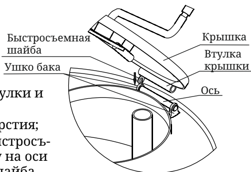
Рисунок 10. Установка крышки бака
