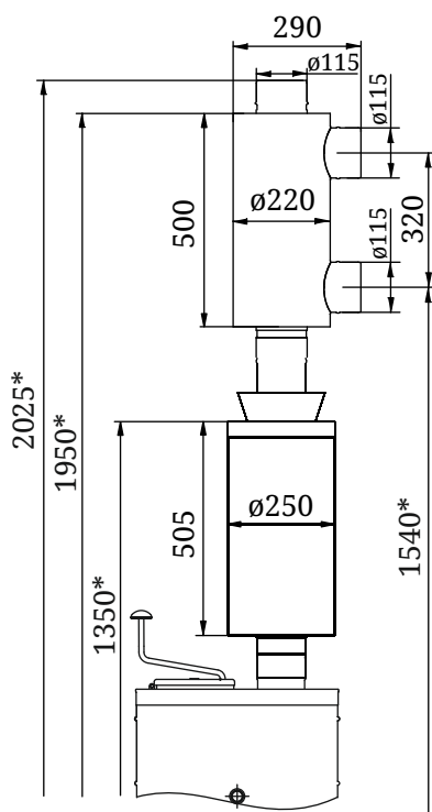
Рисунок 3. Габаритно-монтажные размеры печи-кондиционера модификация «Скоропарка 2012 Баррель»
