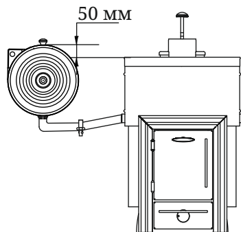
Рисунок 11. Система поддержания уровня воды
