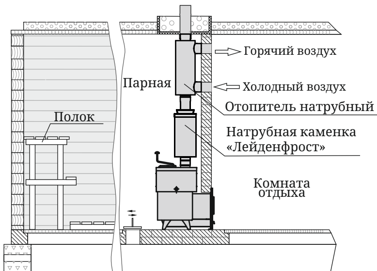
Рисунок 7. Вариант установки отопителя натрубного
