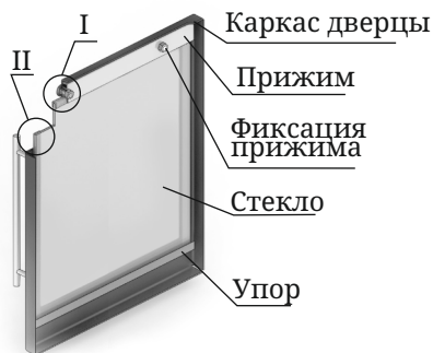
Рисунок 12. Ремонт светорозрачного экрана дверцы модификации «Люмина»
