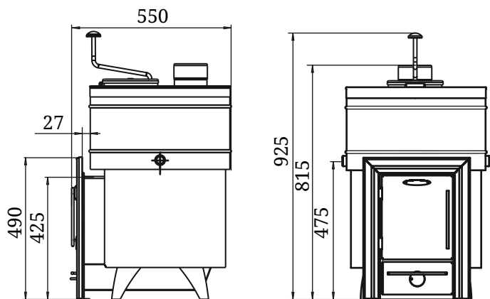
Рисунок 2. Габаритно-монтажные размеры печи «Скоропарка 2012 КТК»
