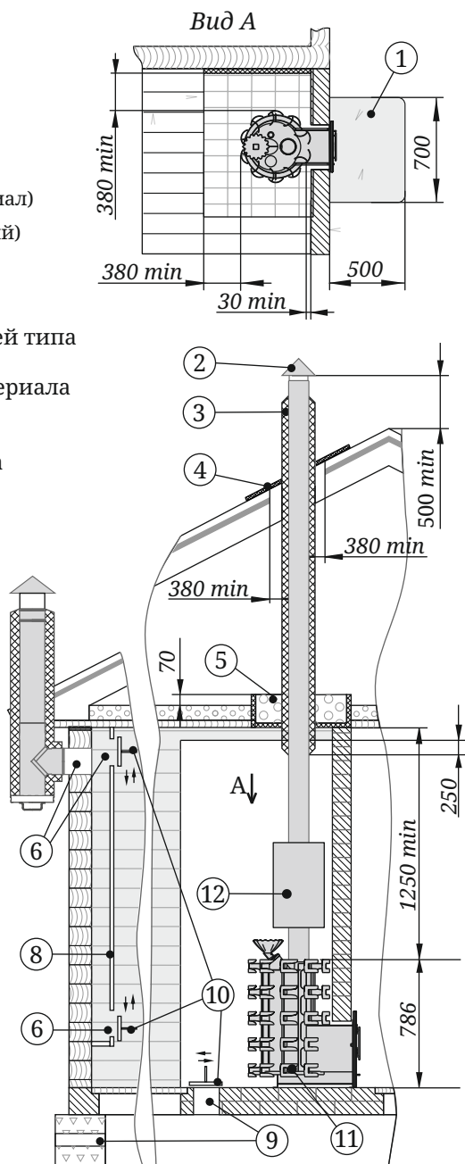
Рисунок 3. Схема монтажа печи
