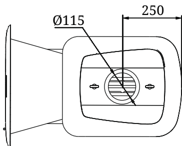
Рисунок 1. Габаритные размеры печи «Каронада Витра»
