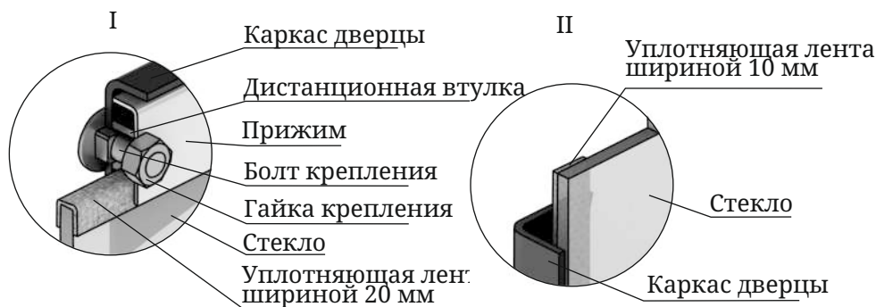
Рисунок 17. Крепление светопрозрачного экрана дверцы модификации «Витра»
