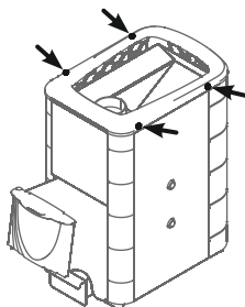
Рисунок 9. Саморезы для демонтажа рамки конвектора печи
