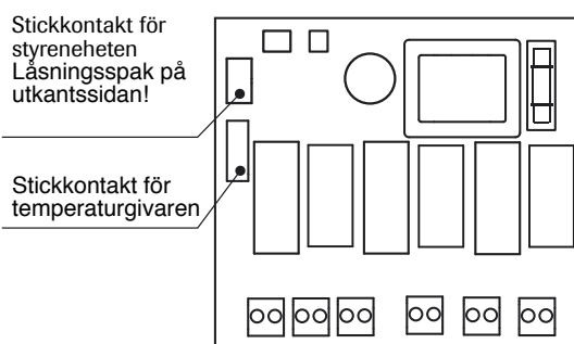
Bild 2.1 Kretskortets anslutningar
