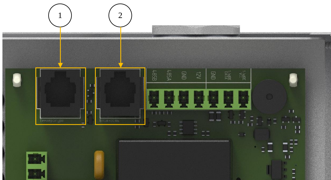
Рис. 29.: Разъёмы для подключения датчиков”.
