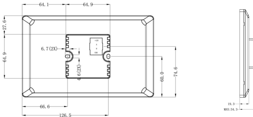
Рис. 21.: Дисплейный модуль. Габаритные размеры.
