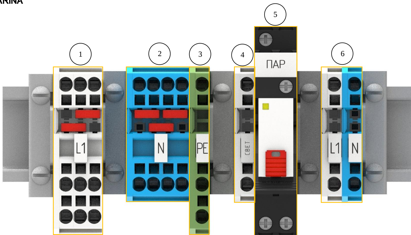
Рис. 8.: “Колодочная сборка”. Однофазная. Вид спереди.
