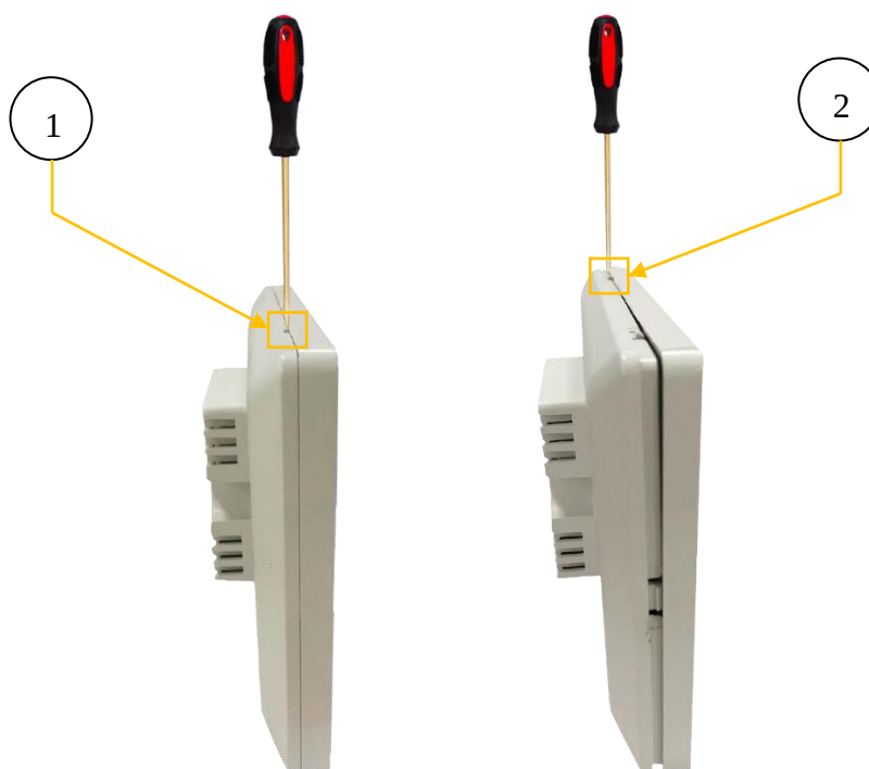
Рис. 22.: Шаг 1. Разъединение панелей дисплея.
