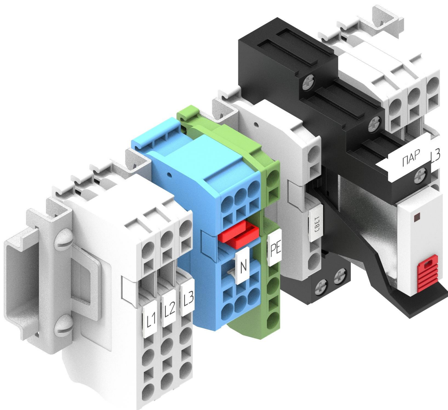
Рис. 7.: “Колодная сборка”. Изометрия.
