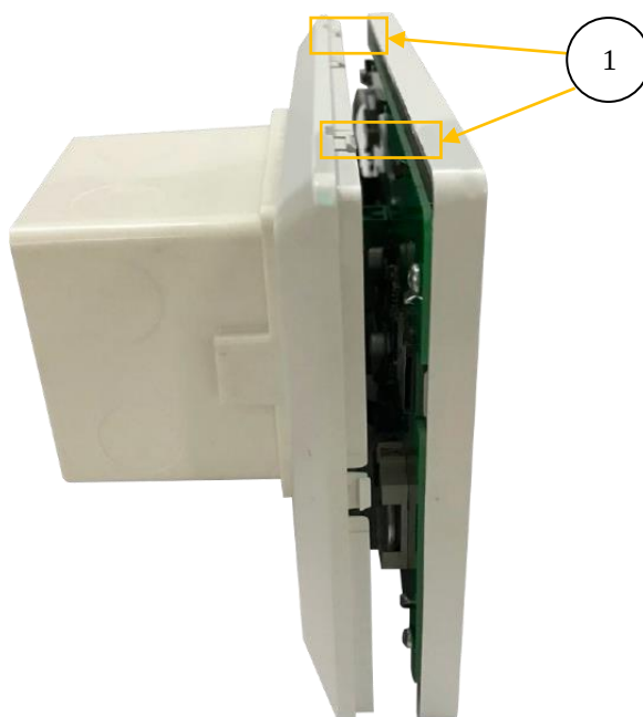
Рис. 27.: Шаг 6. Монтаж передней панели дисплея. 1 – пазы и “язычки”
