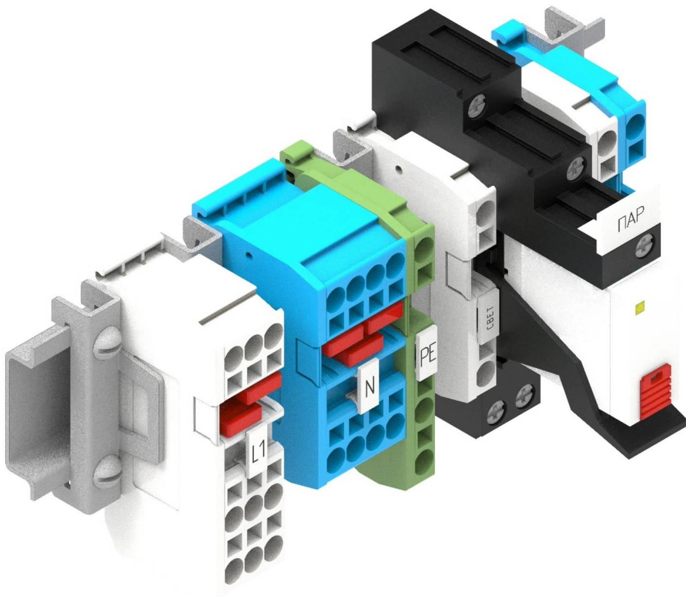
Рис. 9.: “Колодочная сборка”. Однофазная. Изометрия.
