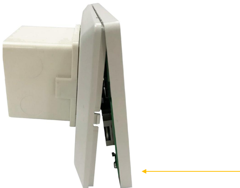
Рис. 28.: Шаг 7. Монтаж передней панели дисплея.
