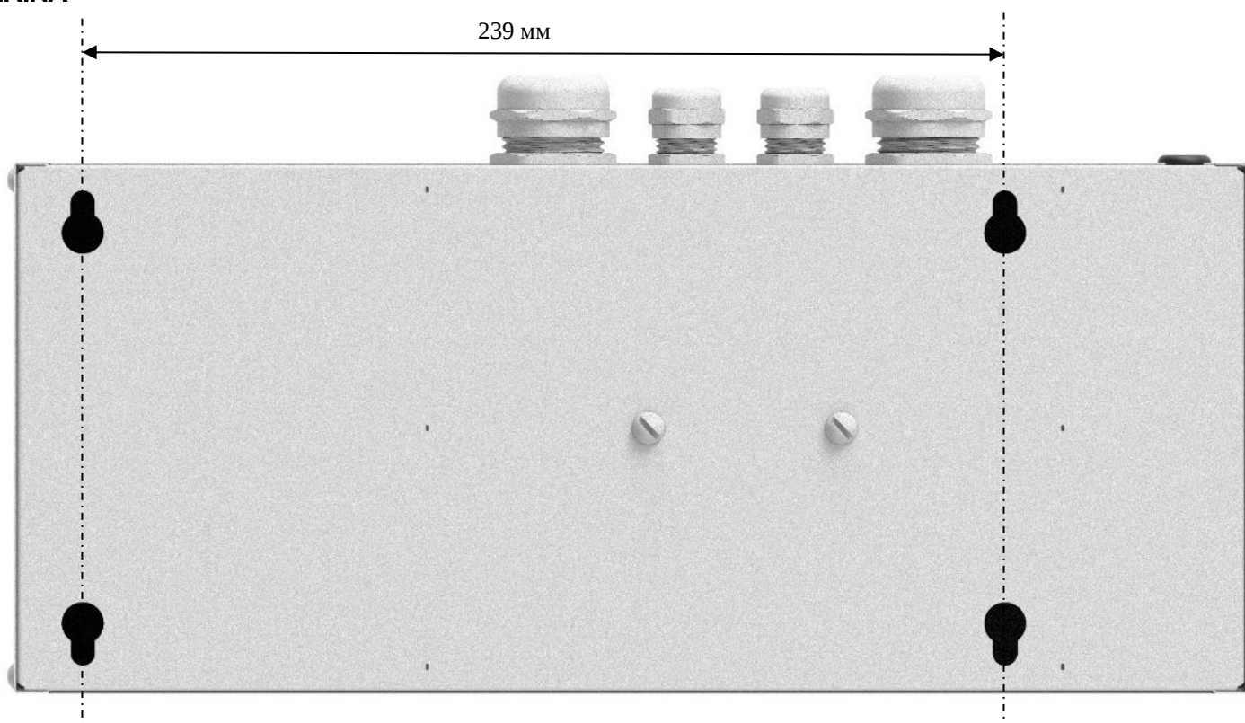
Рис. 18.: Блок мощности. Вид сзади.
