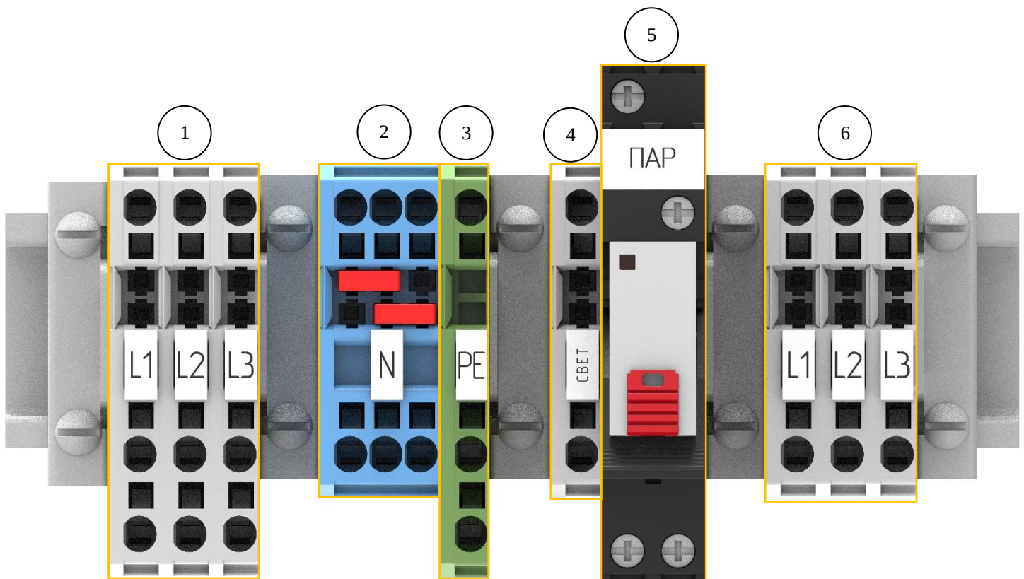
Рис. 6.: “Колодочная сборка”. Трёхфазная. Вид спереди.
