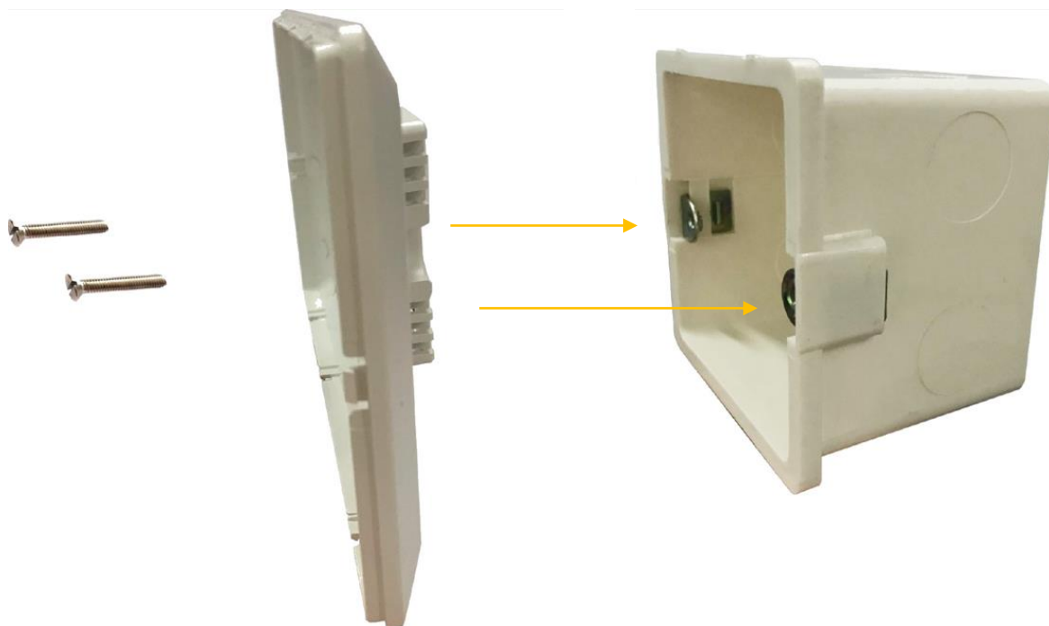
Рис. 24.: Шаг 3: Монтаж задней крышки.
