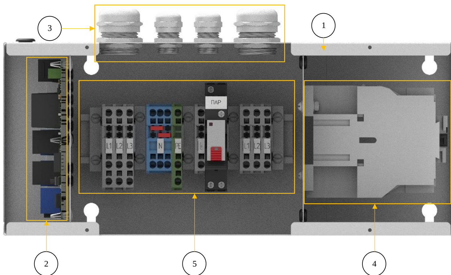
Рис. 4.: “Блок мощности”. Без крышек. Вид спереди.
