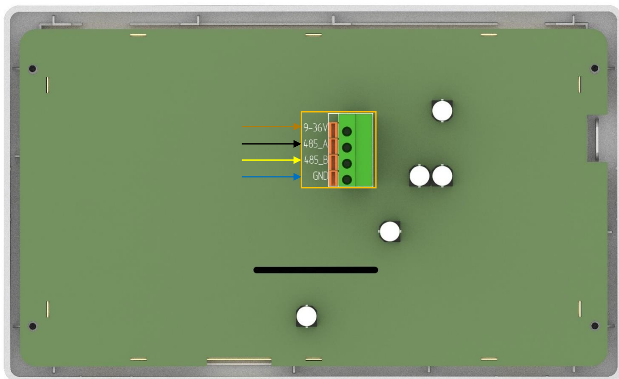
(Рис. 26.: Шаги 4.4.1 - 4.4.4. Подключение дисплейного модуля к “блоку мощности”. Схема расположения подключаемых проводников.)
