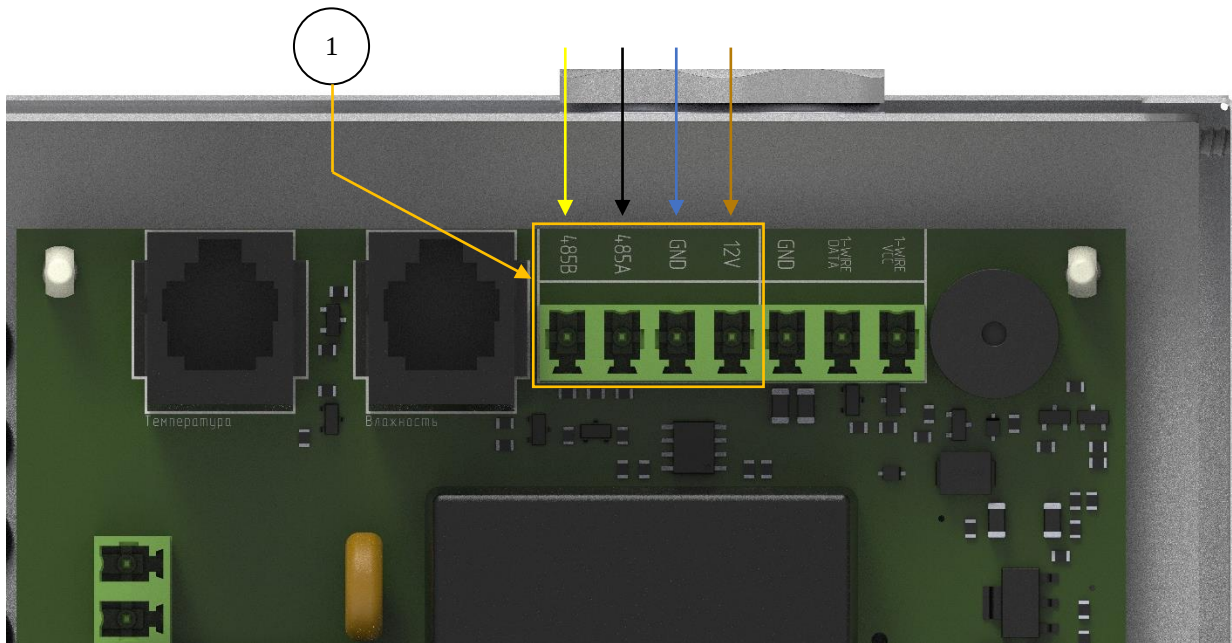
Рис. 25.: Шаги 4.1 – 4.3. Подключение дисплейного модуля к “блоку мощности”.
