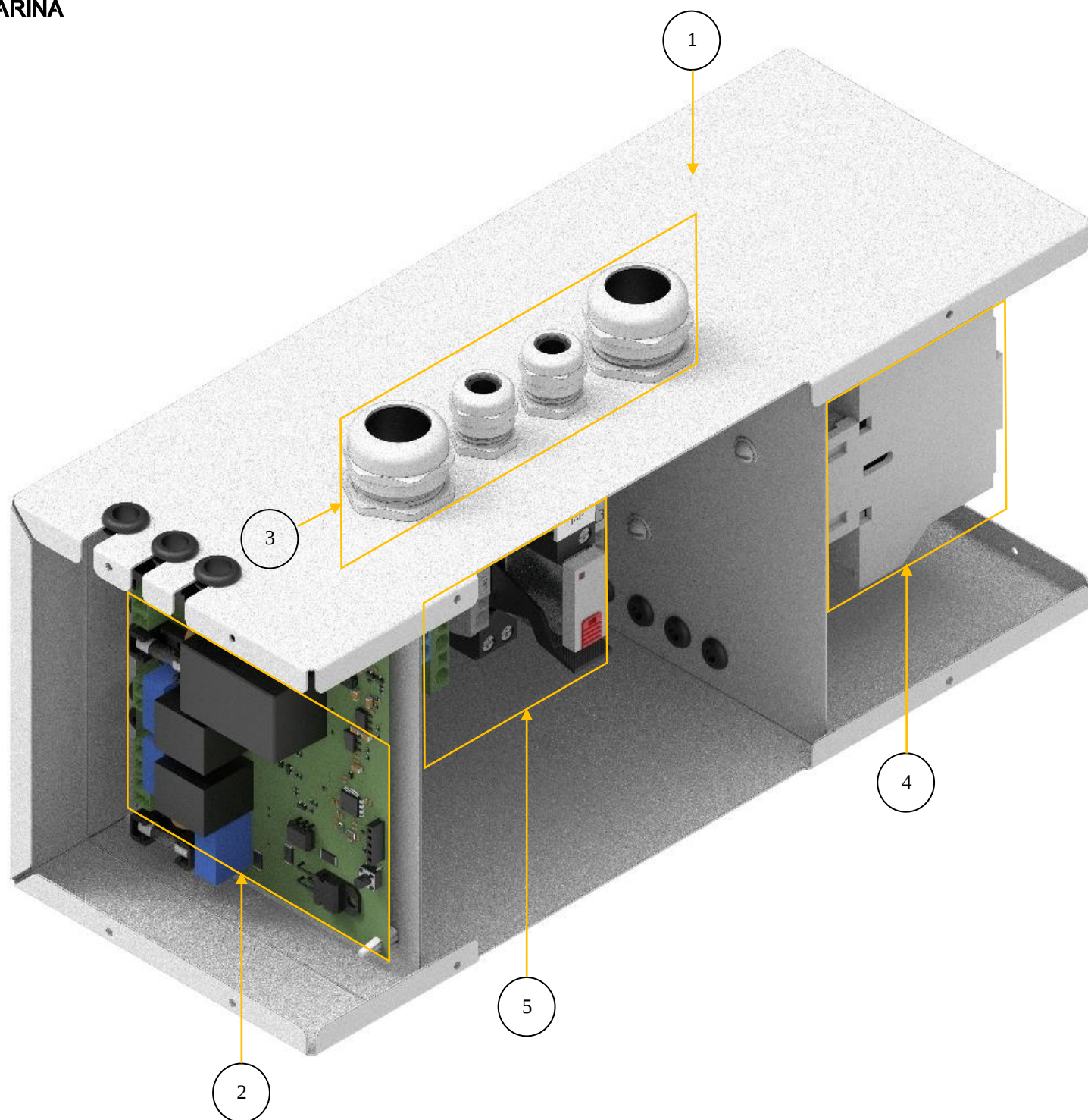
Рис. 5.: “Блок мощности”. Без крышек. Изометрия.
