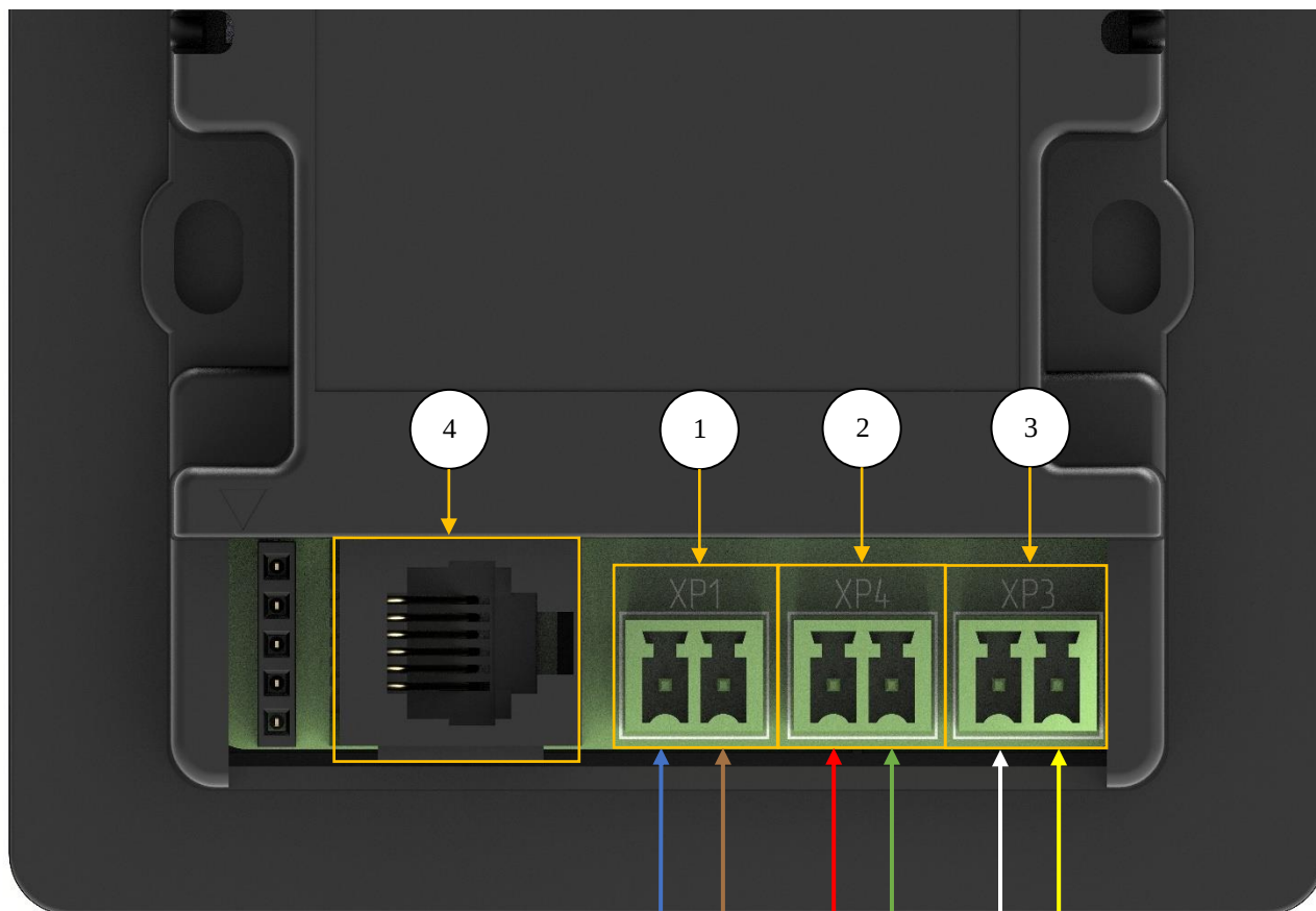
Рис 25.: Подключение дисплейного модуля к блоку мощности.
