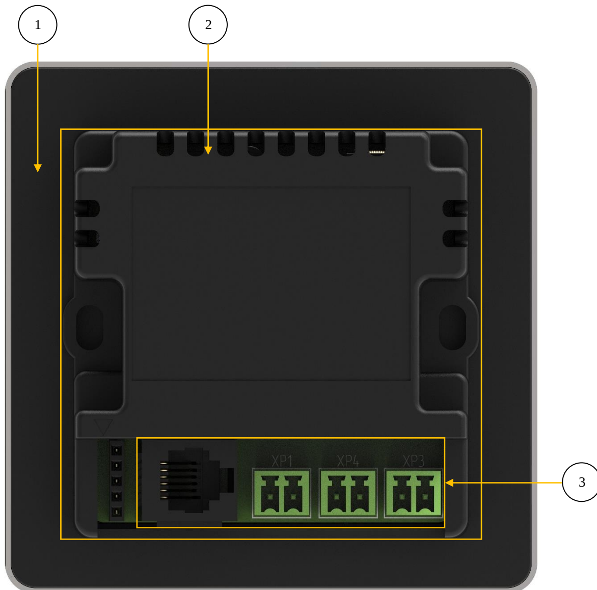
Рис. 12.: Дисплейный модуль. Вид сзади. Взаимное расположение частей модуля: 1 – Задняя крышка, 2 – Разъём для монтажа в подрозетник, 3 – Разъём и колодки для подключения кабелей.
