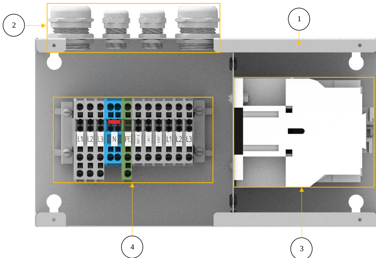
Рис. 4.: “Блок мощности”. Без крышек. Вид спереди.
