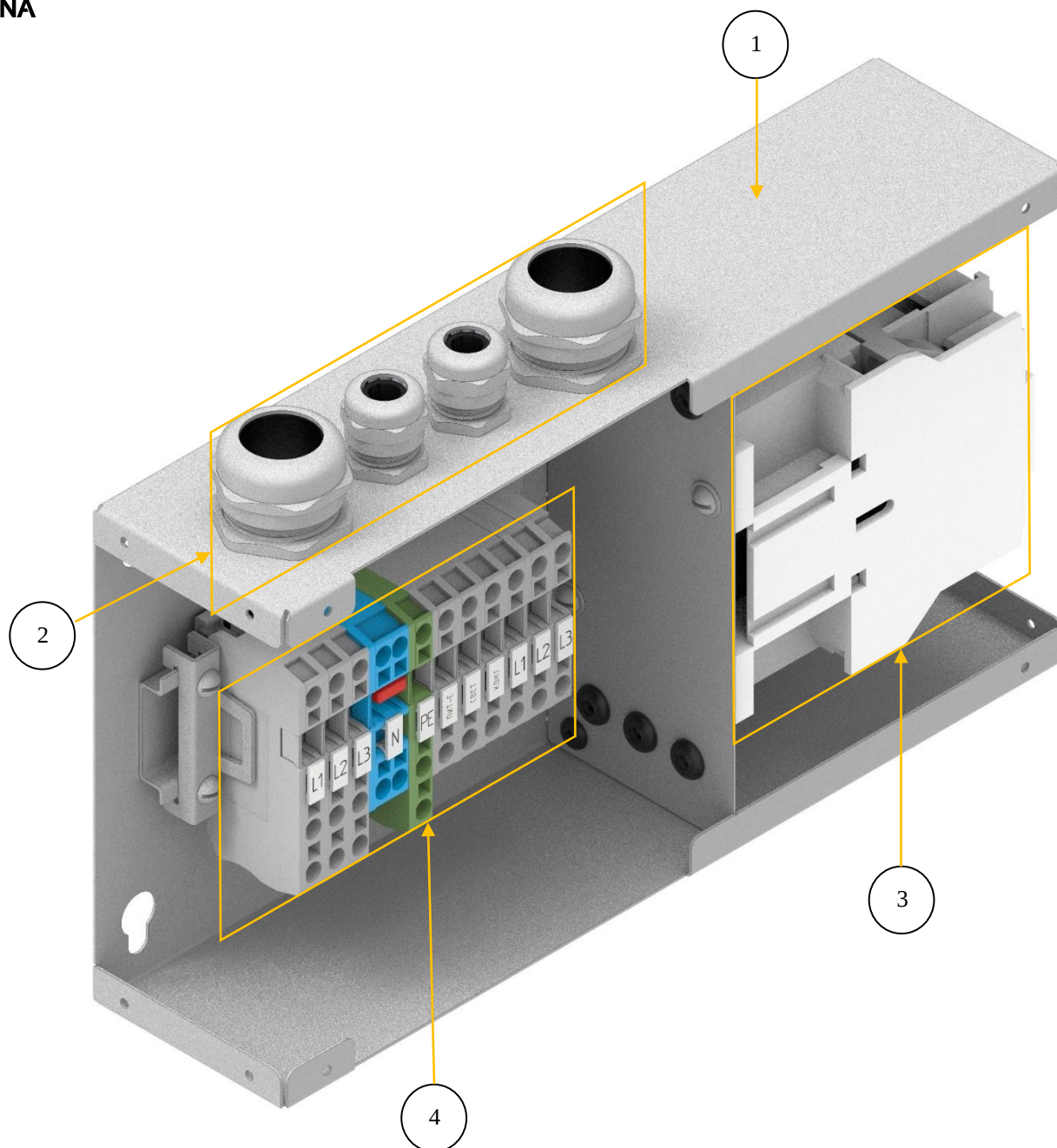
Рис. 5.: “Блок мощности”. Без крышек. Изометрия.
