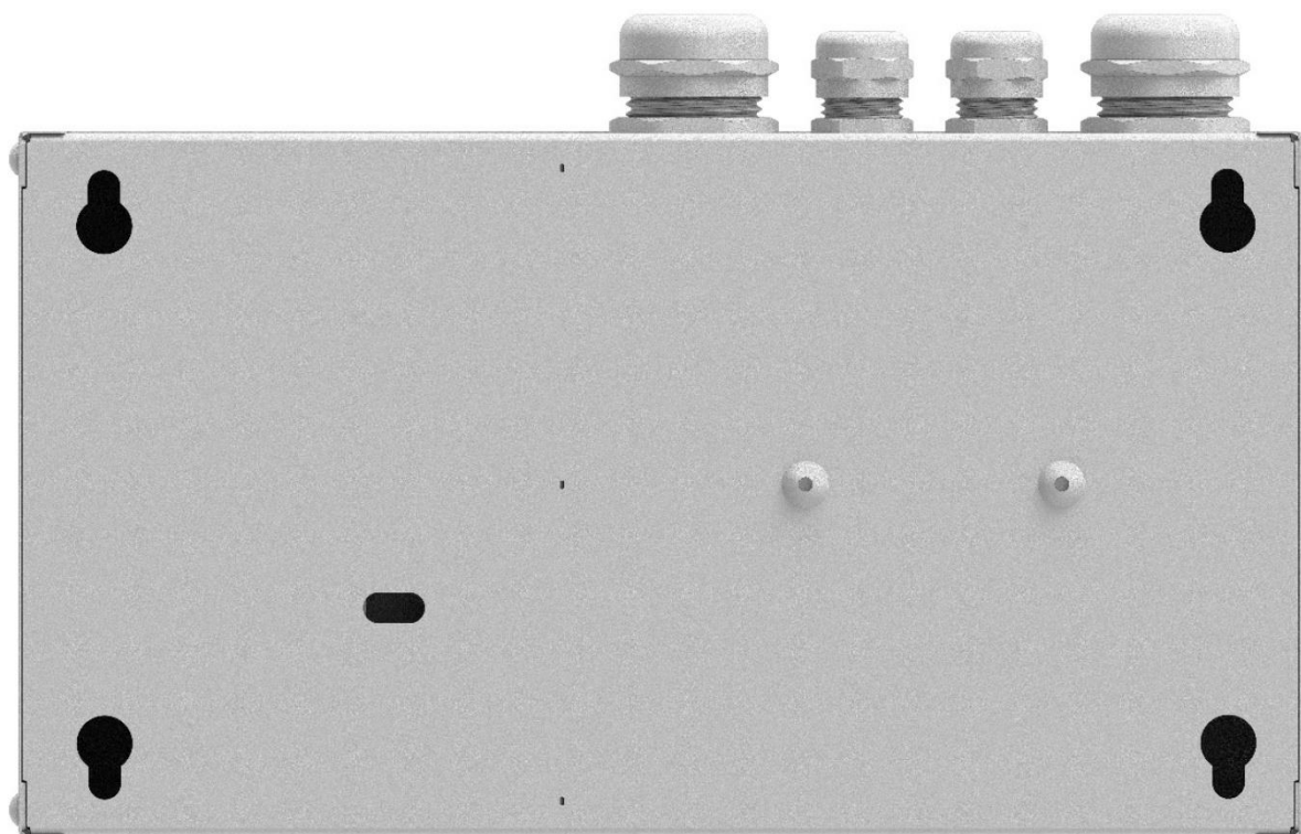
Рис.3.: “Блок мощности”. С крышками. Вид сзади.
