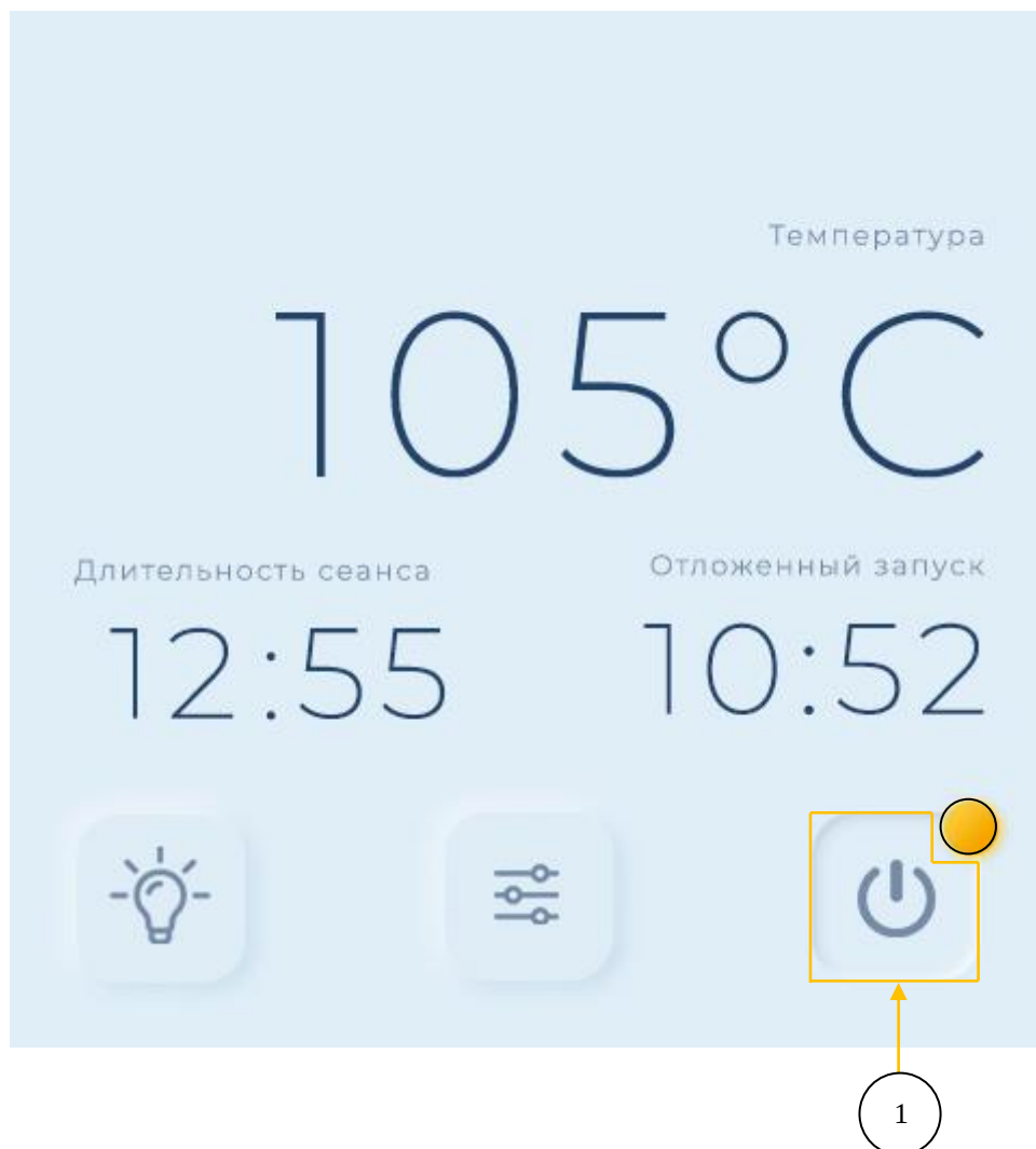
Рис. 39. Взаимное расположение элементов интерфейса “Главной” страницы в режиме отложенного запуска.
