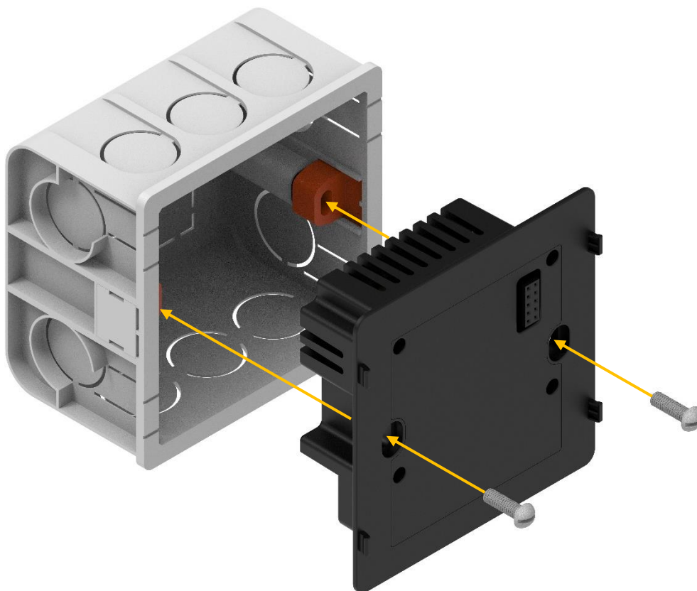
Рис. 26.: Монтаж блока питания / коммутации. Изначальное состояние.
