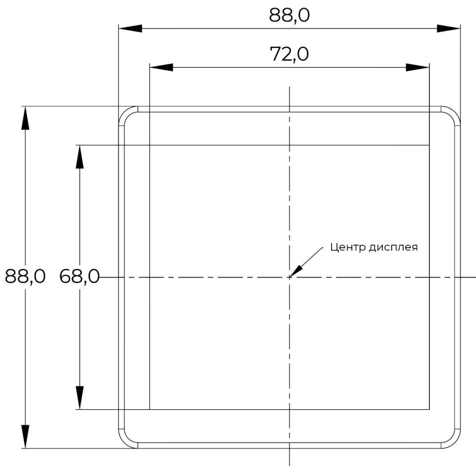
Рис. 21.: Дисплейный модуль. Эскиз. Вид спереди.
