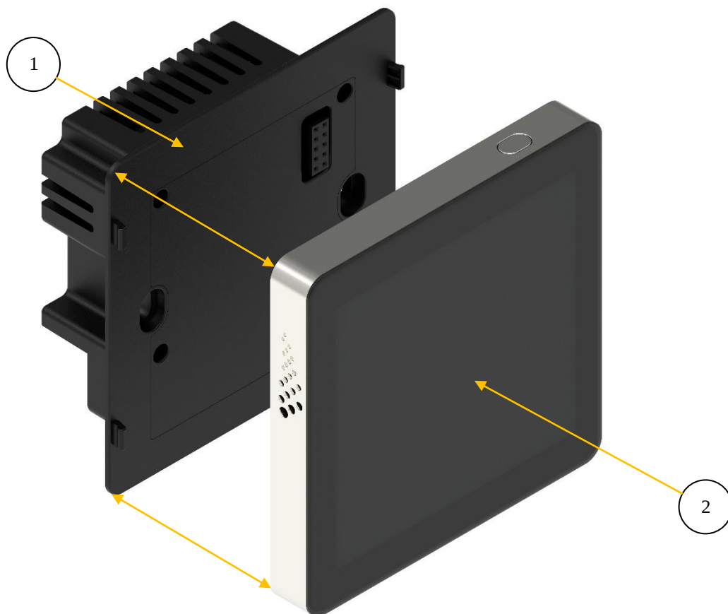
Рис 24.: Дисплейный модуль. Разъединение. Изометрия.
