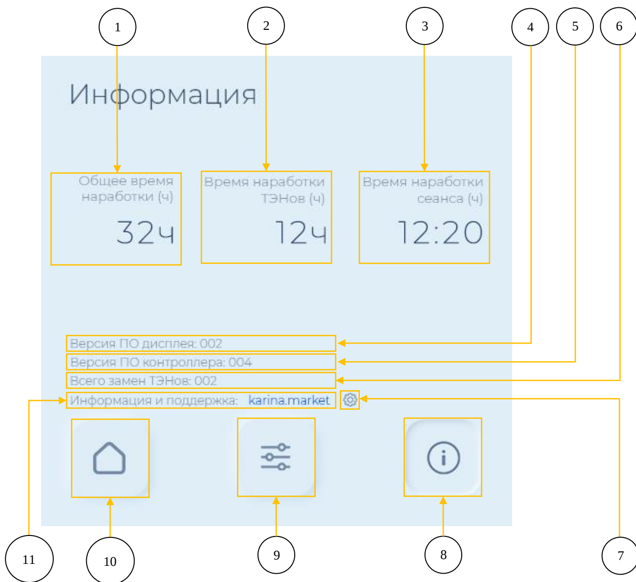
Рис. 34. Взаимное расположение элементов интерфейса “информационной” страницы.
