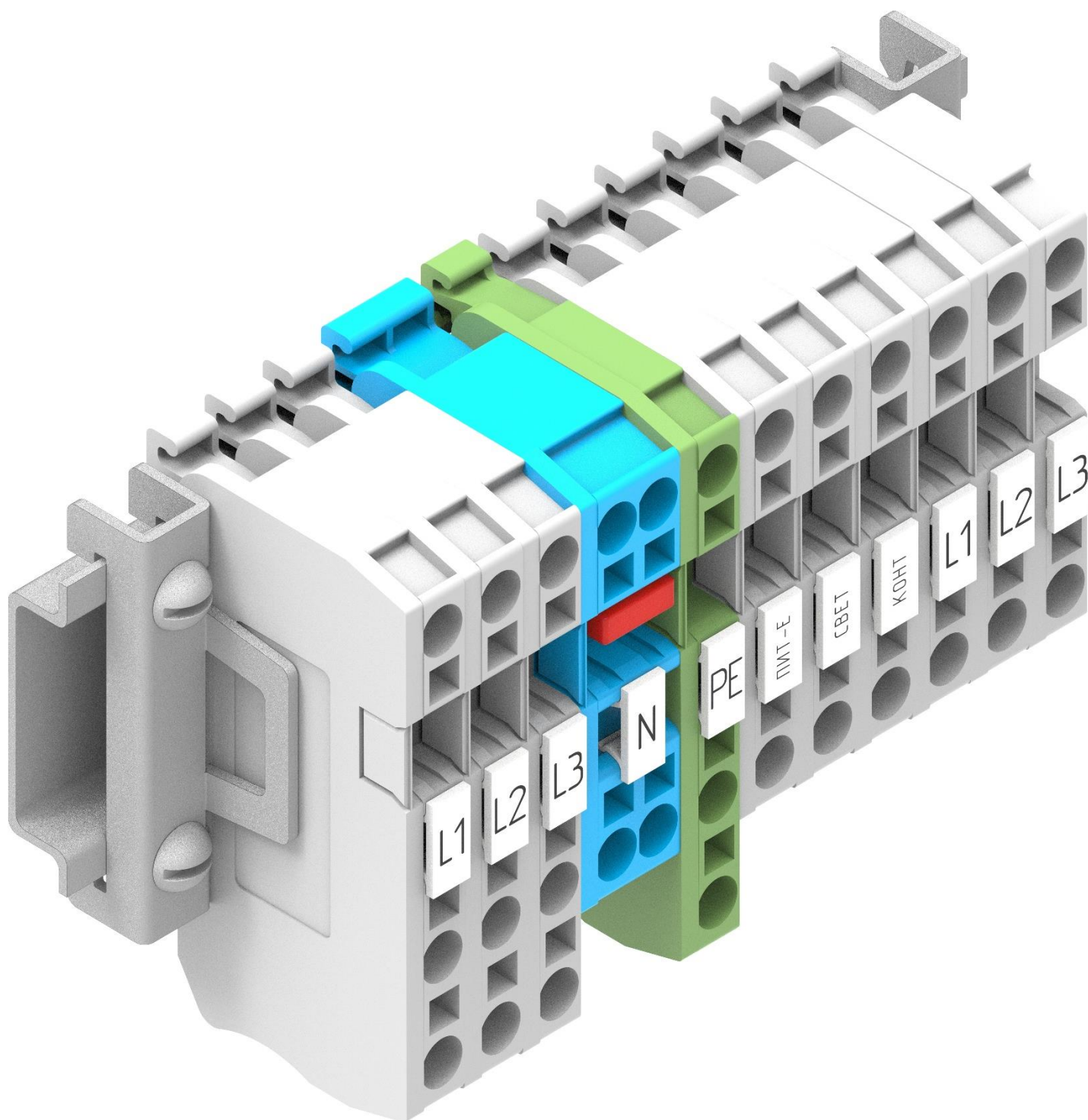
Рис. 7.: “Колодочная сборка”. Изометрия.
