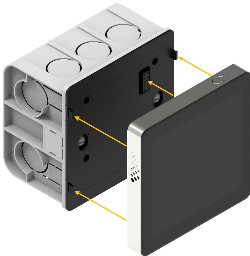
Рис. 28.: Монтаж дисплейного блока. Изначальное состояние.
