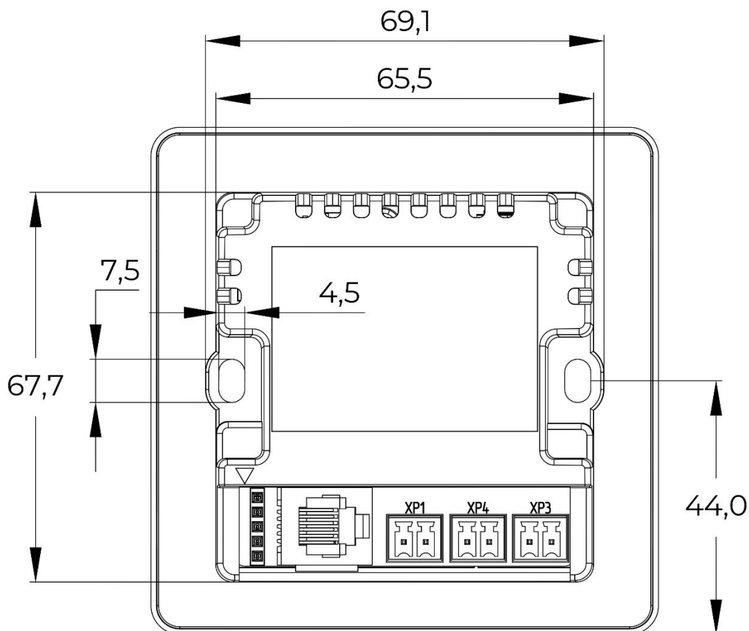
Рис. 22.: Дисплейный модуль. Эскиз. Вид сзади.
