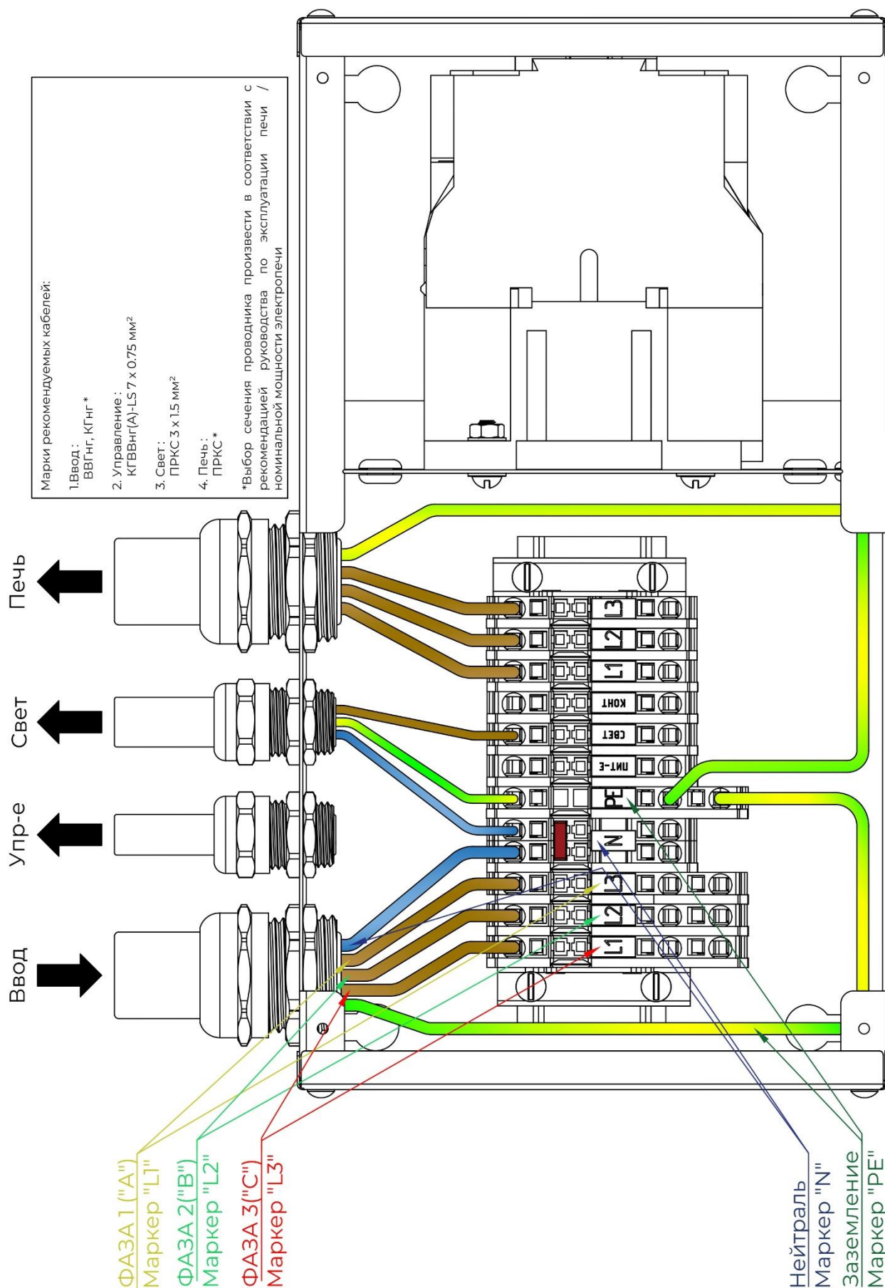
Рис. 17.: Схема расположения подключаемых проводников. Трёхфазный блок. Силовая часть.
