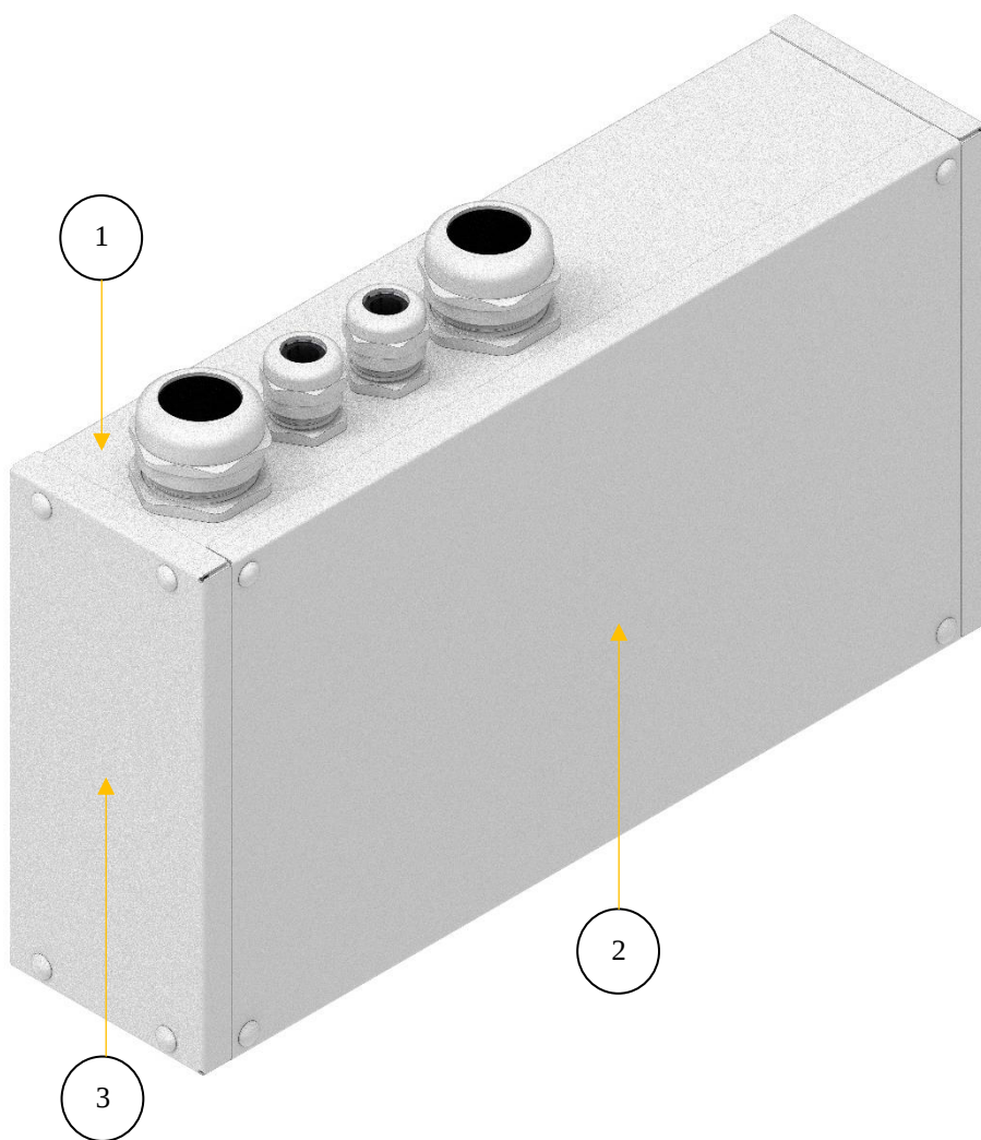
Рис. 2.: “Блок мощности”. С крышками. Изометрия. Взаимное расположение частей модуля: 1 – Двухсекционный корпус, 2 - Крышка передняя, 3 – Крышка торцевая.
