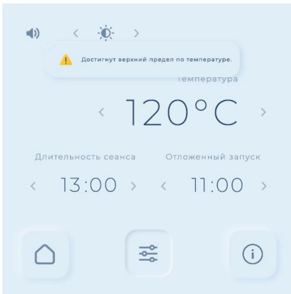
Рис. 38.: Взаимное расположение элементов интерфейса страницы “пользовательские настройки” во время настройки с уведомлением по ограничению температуры.
