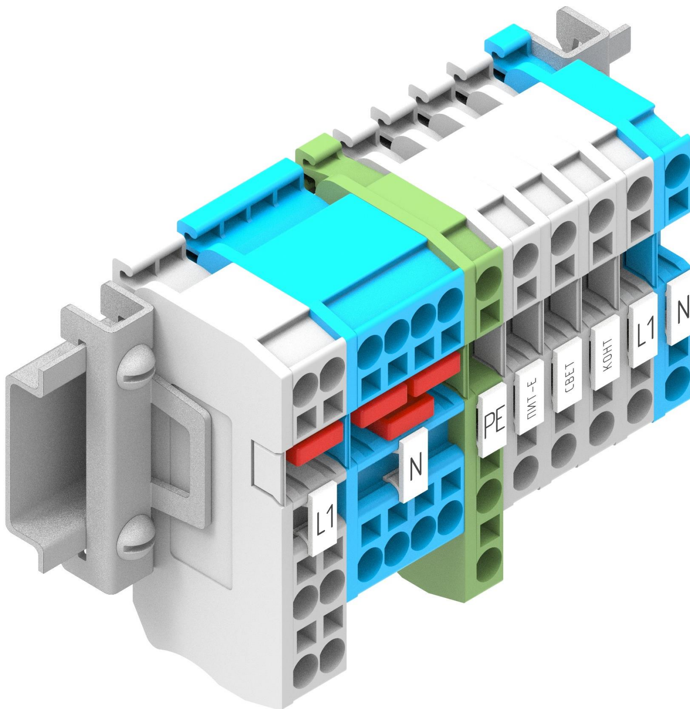
Рис. 9.: “Колодочная сборка”. Однофазная. Изометрия.
