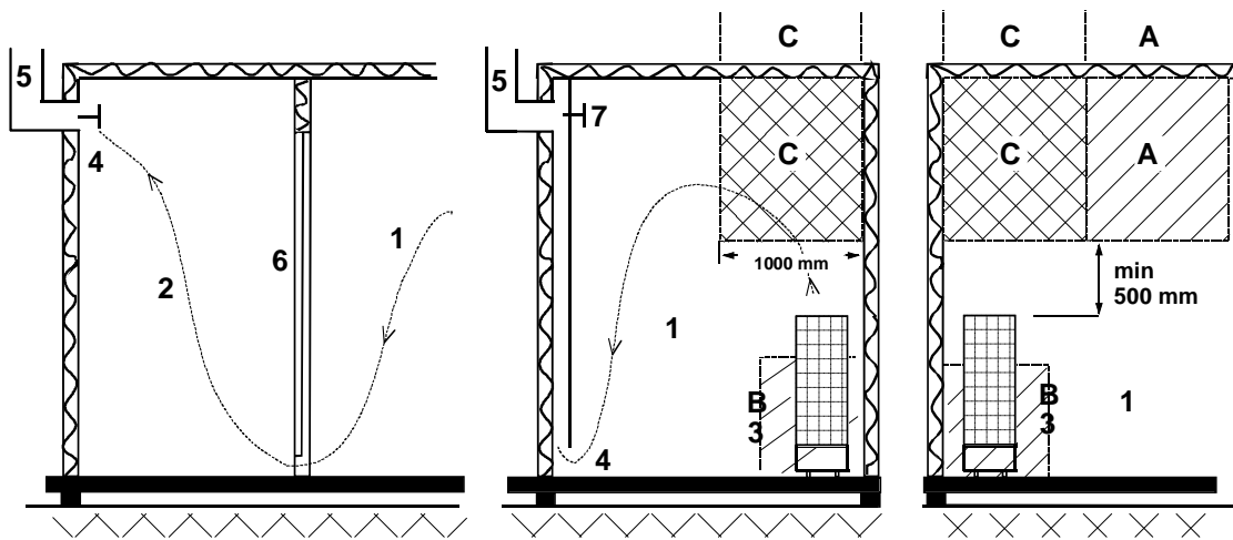
Bild 10 Empfohlene Belüftung des Saunaraums
