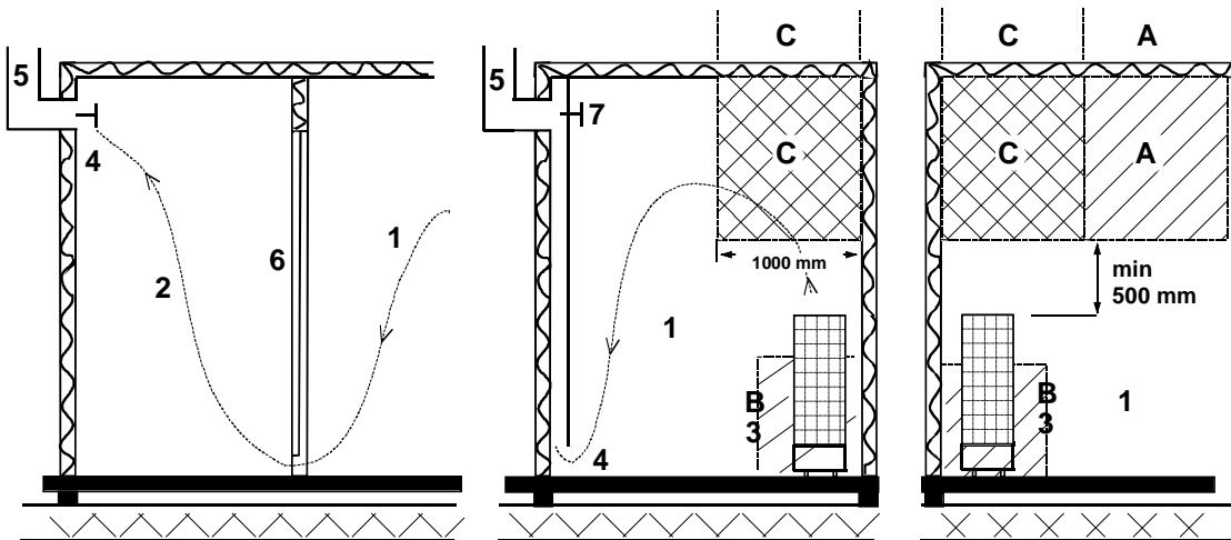
Joonis 10 Lavaruumi soovitatav ventilatsioon
