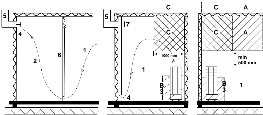
Figura 10 Ventilación recomendada para la sauna
