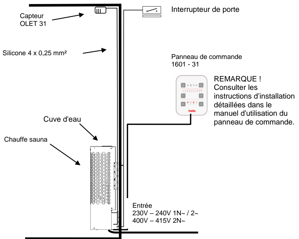
Figure 11 Du principe de fonctionnement
