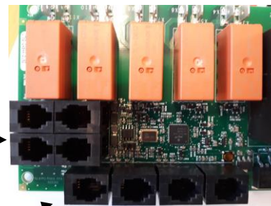
Obrázek 8 . . Pořadí konektorů RJ 10. Senzor, dveřní spínač, dálkové ovládání, další NTC
