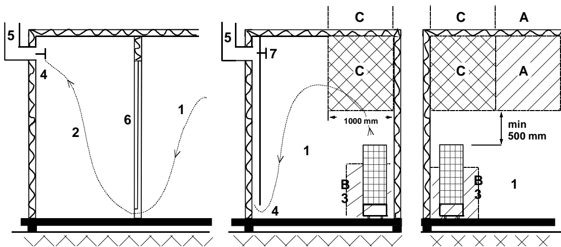
Rysunek 10 Zalecana wentylacja kabiny sauny
