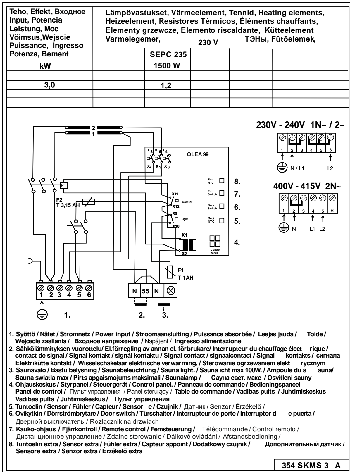
Joonis 9 Saunakerise ühenduste skeem
