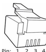
Konnektori RJ10 kontaktide paigutus
