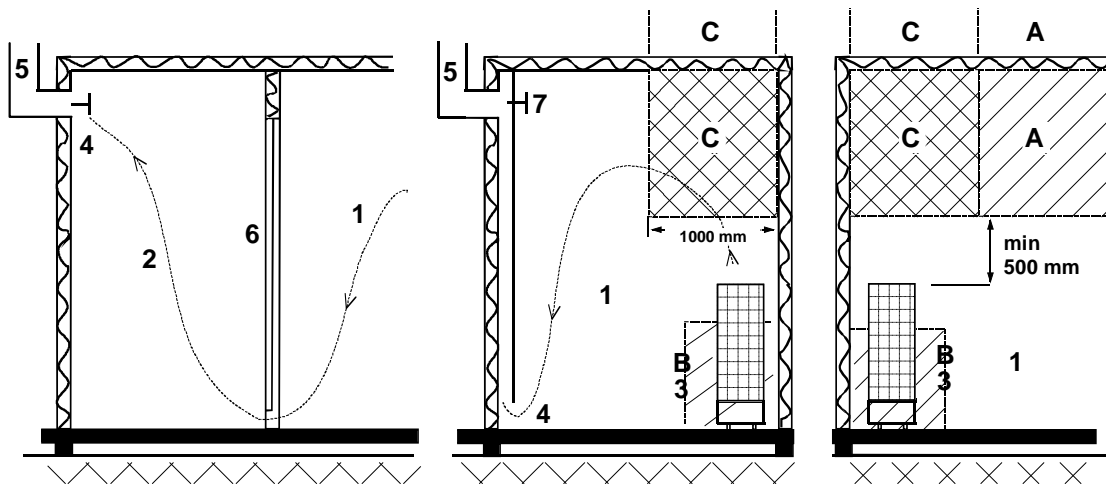
Obrázek 10 Doporučené větrání saunové kabiny
