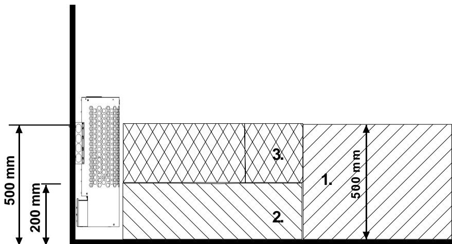
Bild 7 Placering av kopplingsdosa
