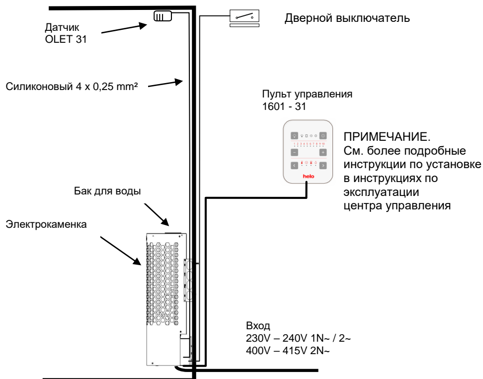
Рис 11 Принципиальная схема
