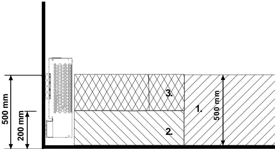
Kuva 7 Kytkentärasian sijoituspaikka
