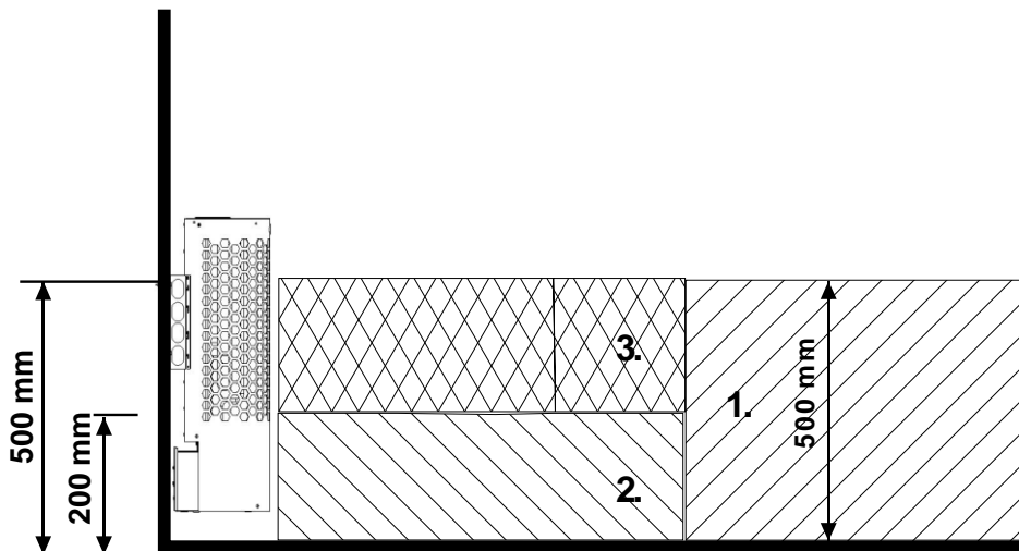
Obrázek 7 Umístění rozvaděče
