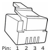
Disposition des broches sur un connecteur RJ10
