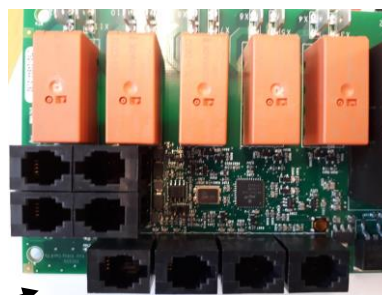
Joonis 8 . RJ 10 -konnektorite järjestus. Sensor, ukselülit, kaugjuhtimisseade, täiendav NTC
