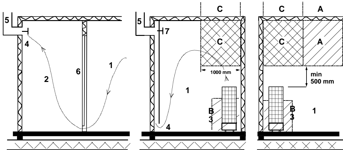
Bild 10 Rekommenderad ventilation i bastun
