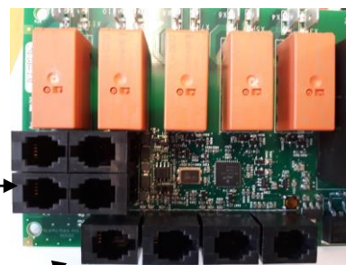
Rysunek 8 . Kolejność złączy RJ 10. Czujnik, przełącznik drzwiowy, sterowanie zdalne, dodatkowe NTC
