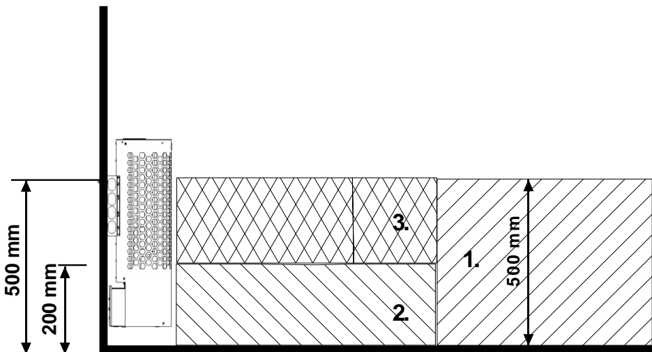
Joonis 7 Ühenduskarbi asukoht
