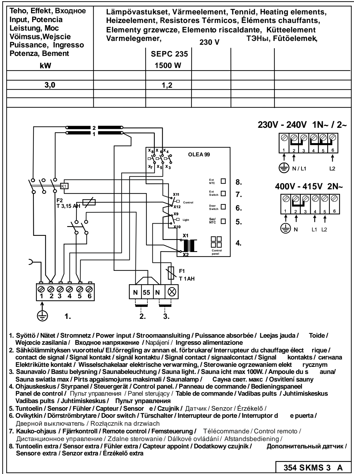
Рис 9 Схема электрических соединений
