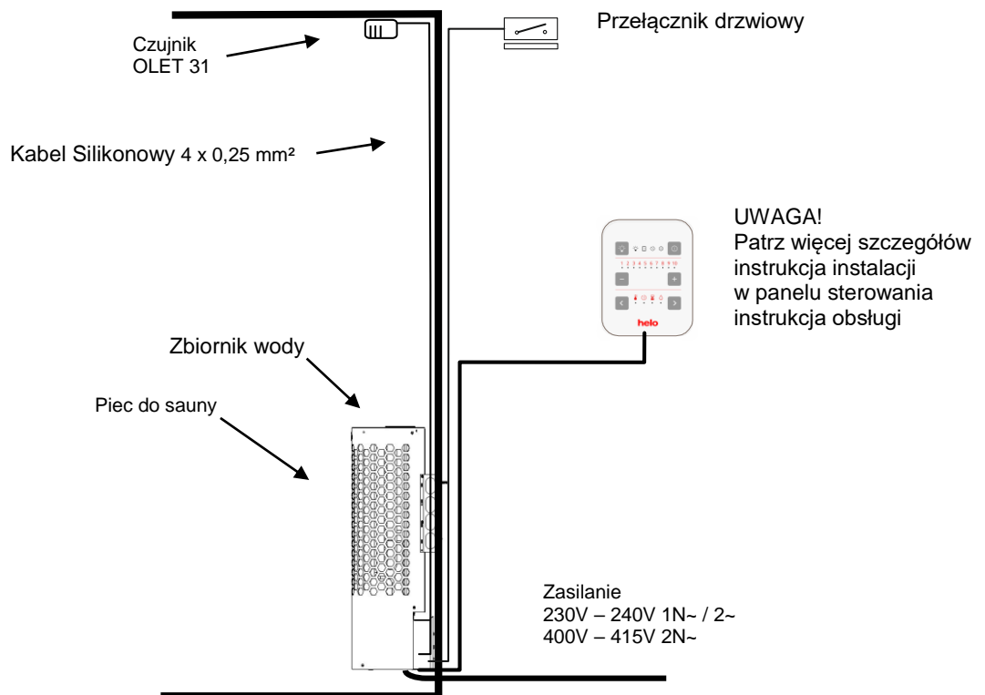
Rysunek 11 Rysunek poglądowy
