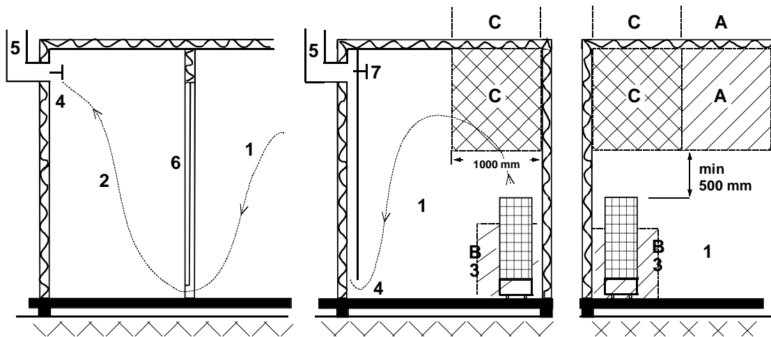
Figure 10 Recommandations à propos de la ventilation de la cabine de sauna
