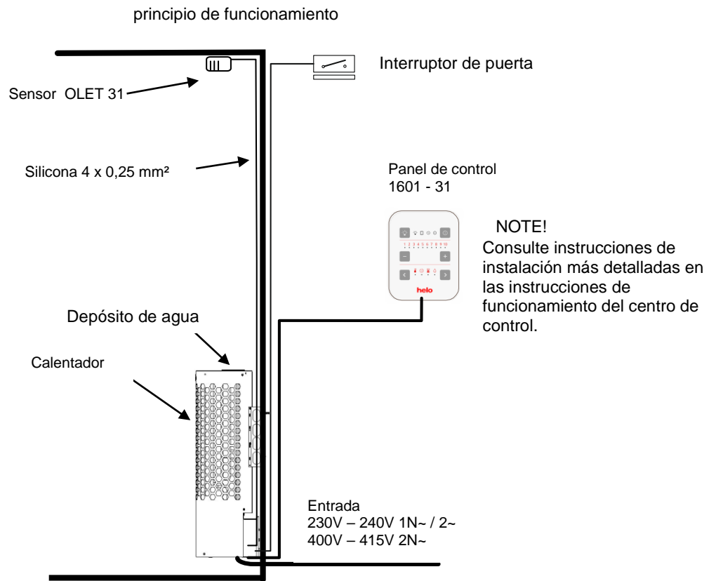
Figura 11 Principio de funcionamiento.
