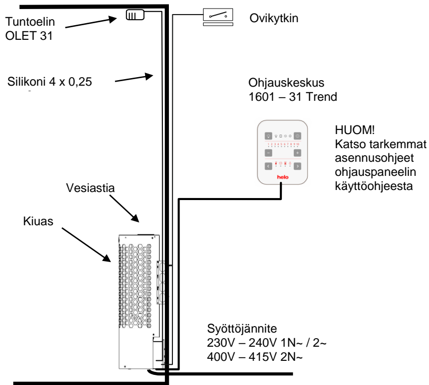
Kuva 11 Periaatekuva kytkennästä
