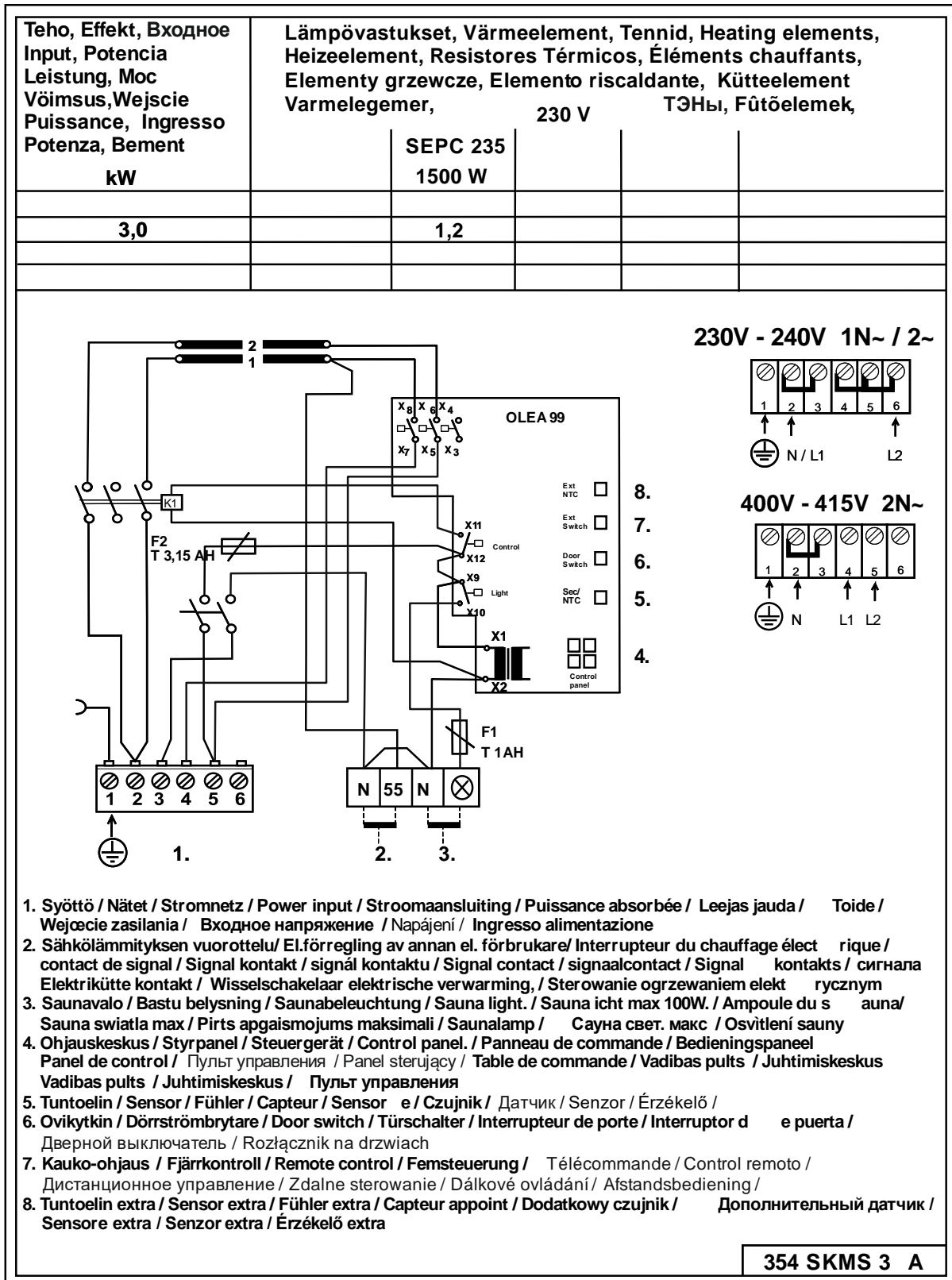
Figura 9 Diagrama de conexiones
