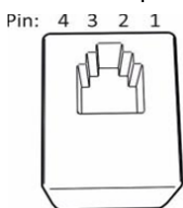
Trükkplaadi konnektori RJ10 kontaktide paigutus
