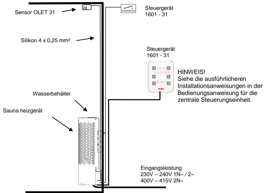
Bild 11 Prinzipbild mit Steuergerät 1601-31 (RA – 31 Trend )
