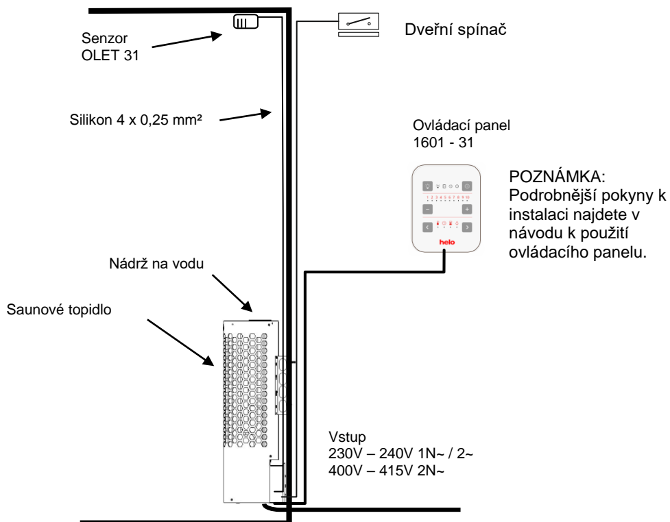
Obrázek 11 Schéma zapojen
