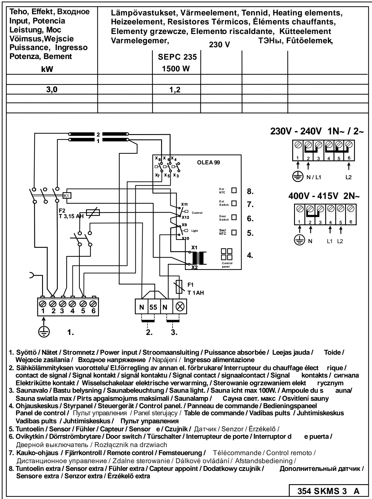
Bild 9 Schaltdiagramm
