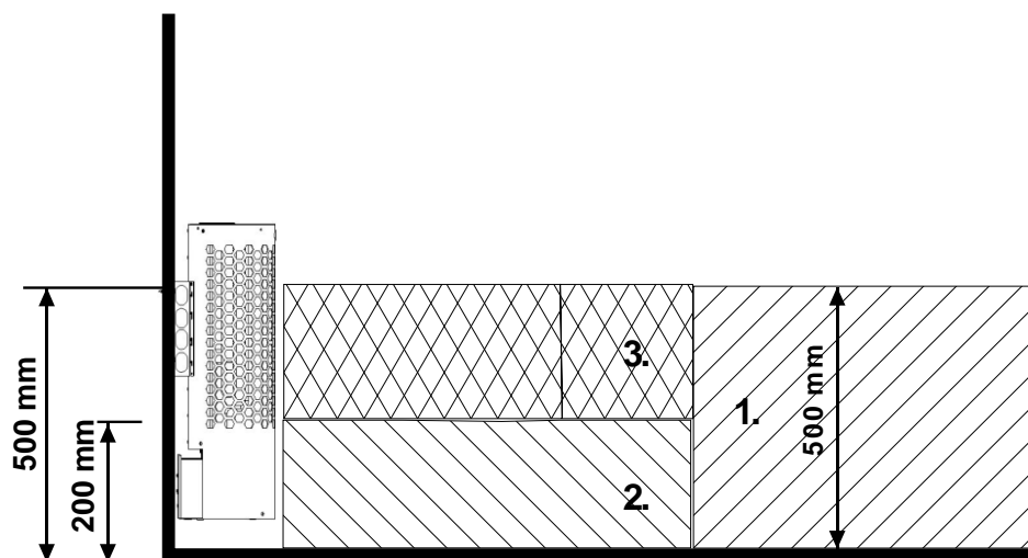
Rysunek 7 Lokalizacja skrzynki rozdzielczej
