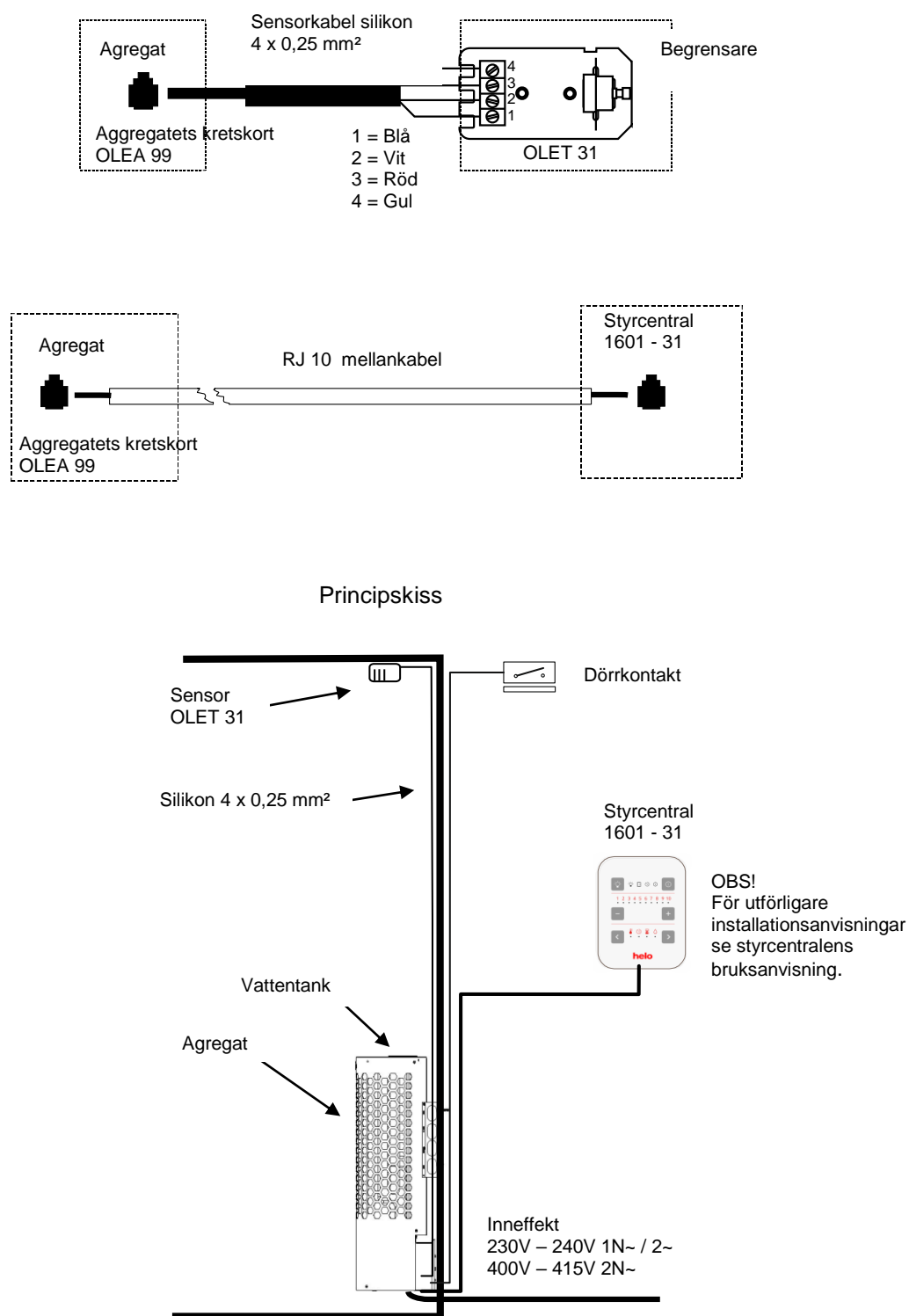
Bild 11 Principskiss
