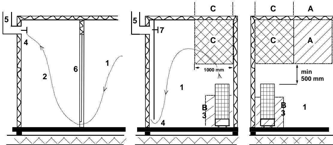
Kuva 10 Suositeltava ilmanvaihto saunassa
