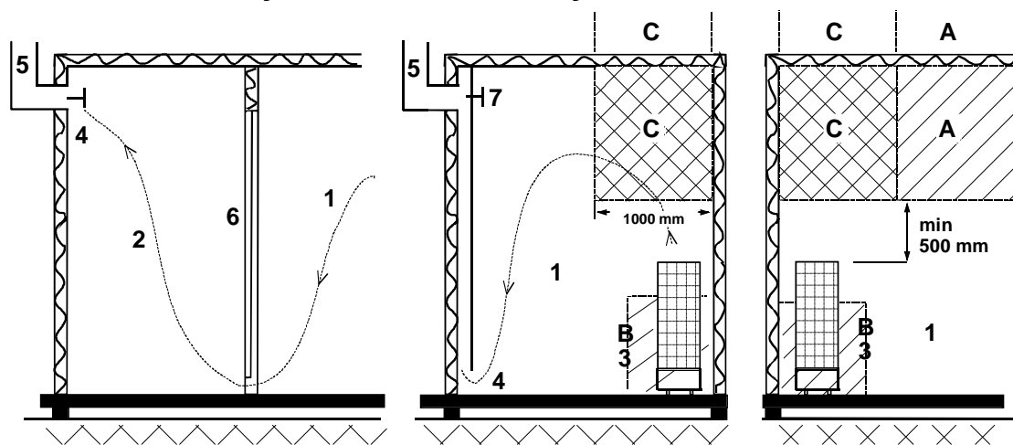
Рис 10 Рекомендуемая вентиляция сауны
