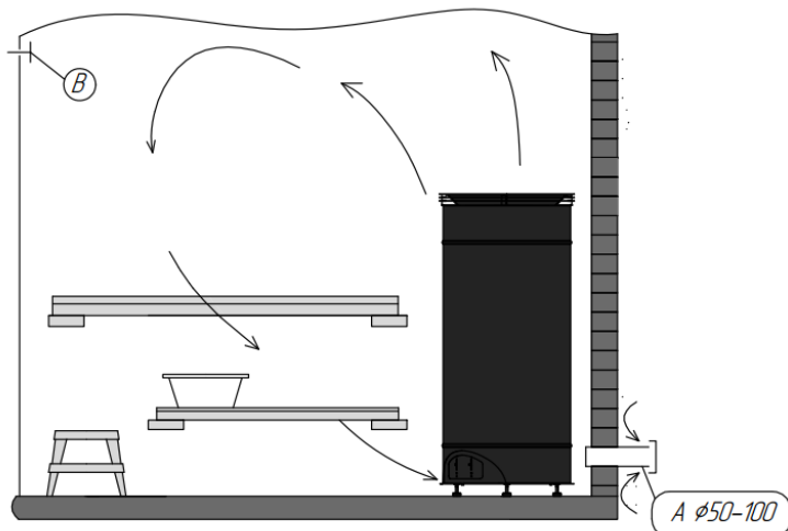
Рисунок 1. Естественная вентиляция
