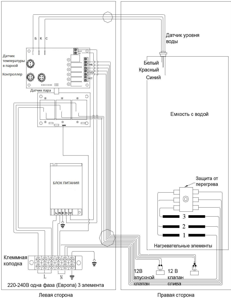
Рисунок 10. Электромонтажная схема ST45-P и ST60P
