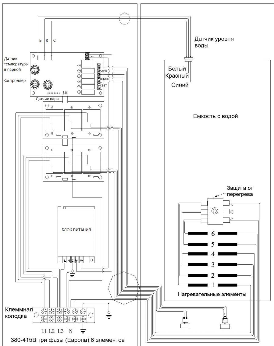
Рисунок 11. Электромонтажная схема ST-90P, ST-120P
