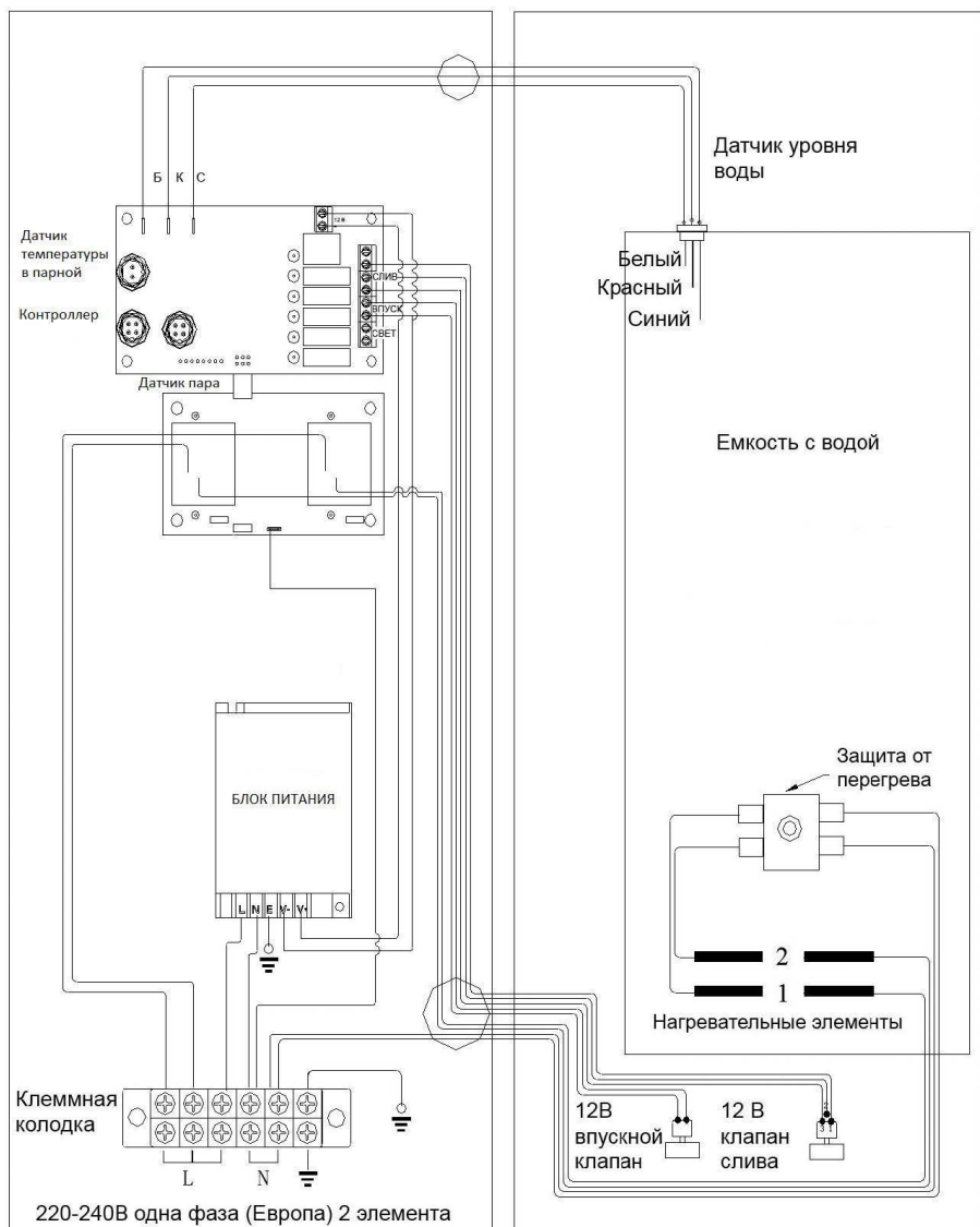
Рисунок 9. Электромонтажная схема ST-30P
