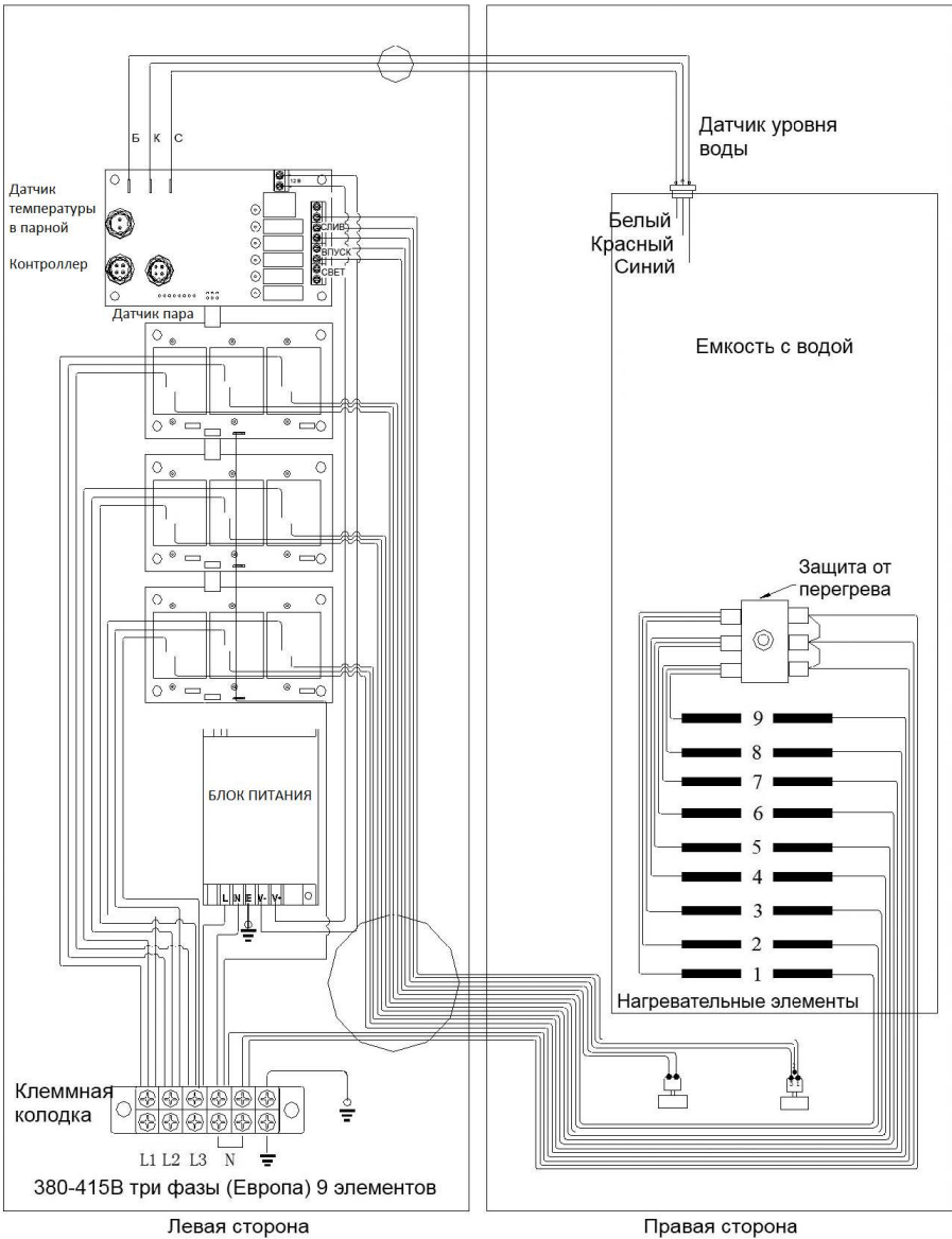
Рисунок 12. Электромонтажная схема ST-150P, ST-180P, ST-225P, ST-240
