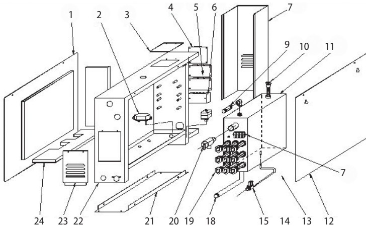
Рисунок 1. Конструкция парогенератора
