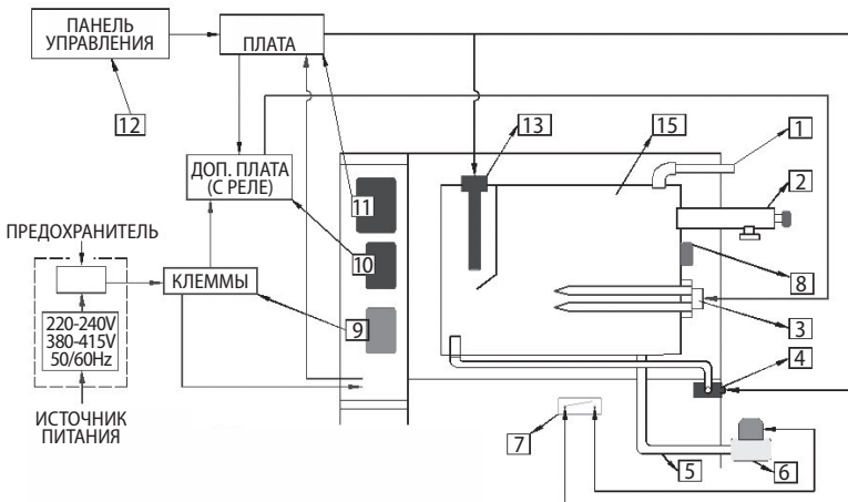
Рисунок 2. Принцип работы парогенератора
