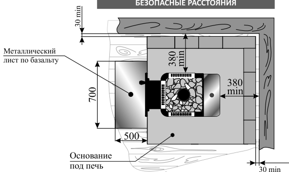
БЕЗОПАСНЫЕ РАССТОЯНИЯ
