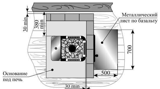
БЕЗОПАСНЫЕ РАССТОЯНИЯ
