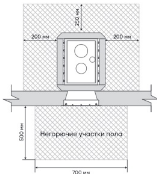
Рис. 2 Размеры негорючего или защищенного участка пола
