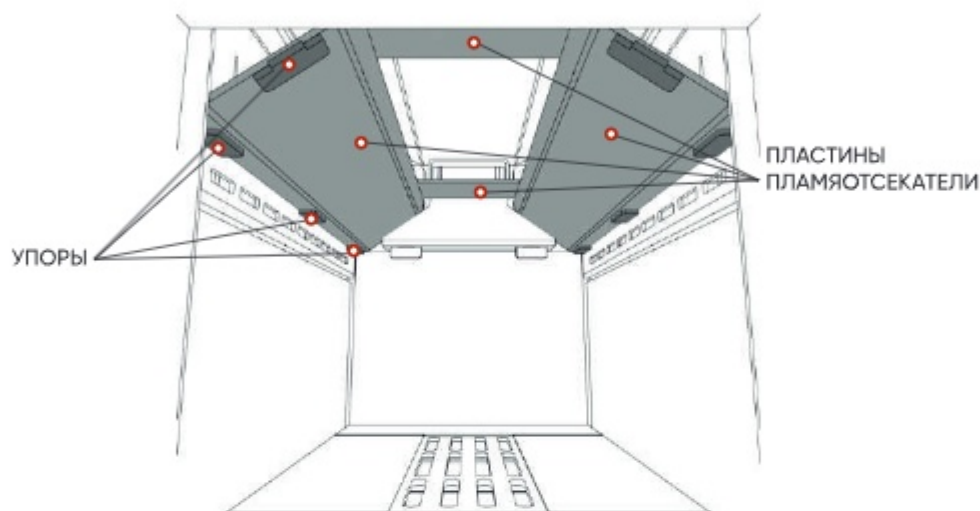
Рис. 10 Пластины пламяотсекатели
