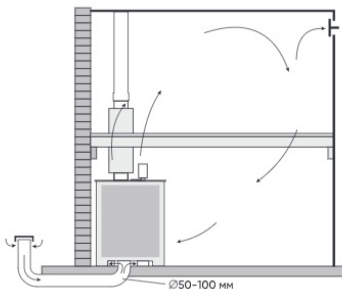
Рис. 6 Естественная вентиляция
