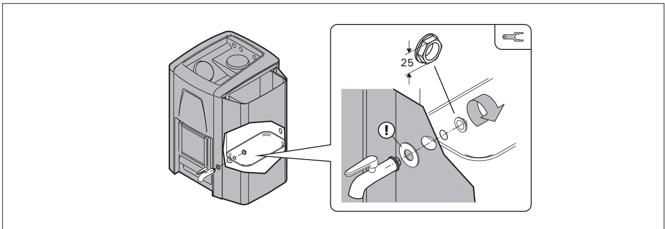
Рисунок 17. Установка крана резервуара для воды
