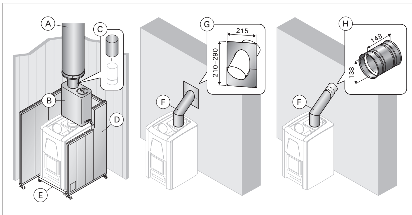
Рисунок 19. Дополнительные принадлежности (все размеры приведены в миллиметрах)
