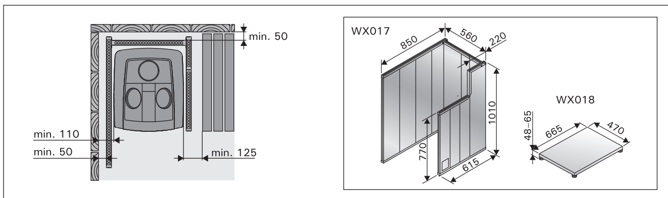
Рисунок 11. Защитные обшивки и основания Harvia (все размеры приведены в миллиметрах)
