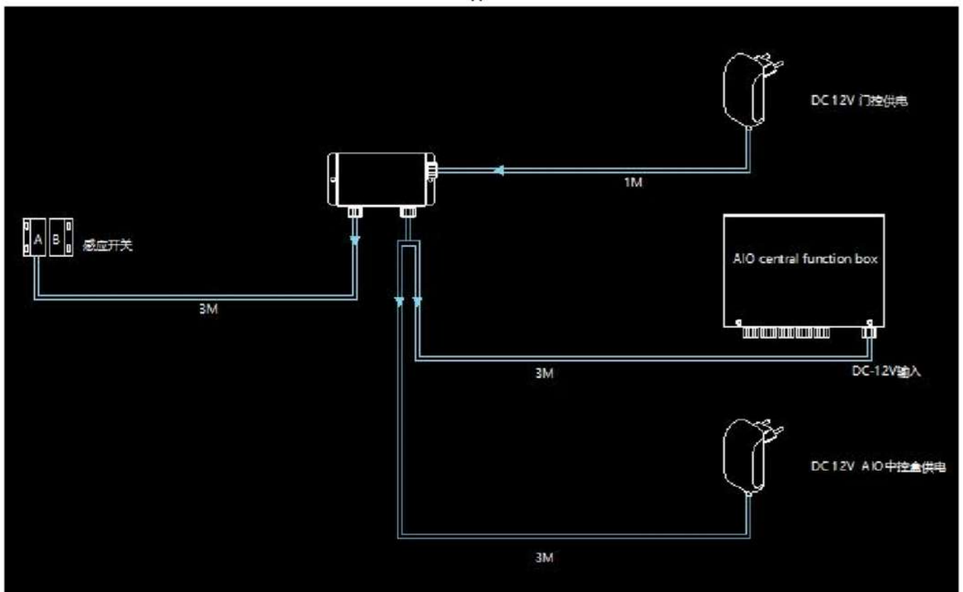
Схема подключения:
